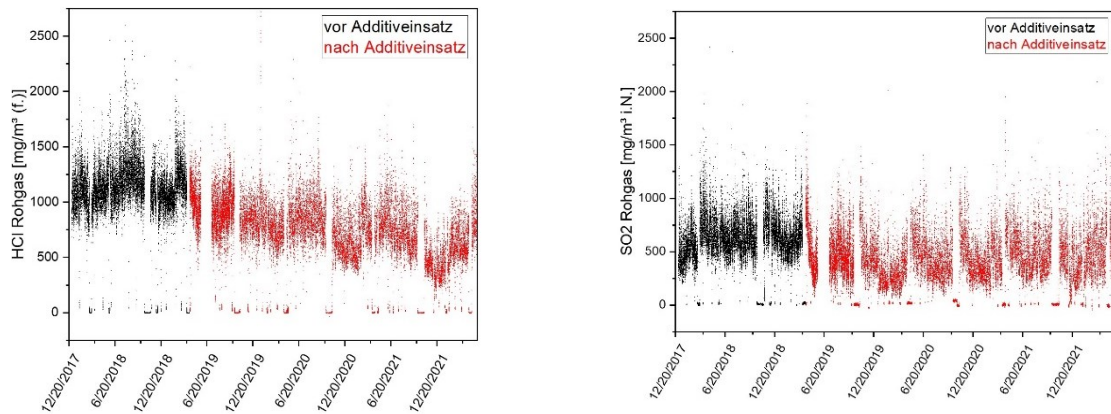
Abbildung 88: MVV Gersthofen (a) HCl- und (b) \text{SO}_2 -Rohgaswerte (Eine-Stunde-Mittelwerte) für die Zeiträume Januar 2018 bis Mai 2022, Additiveinsatz ab April 2019
