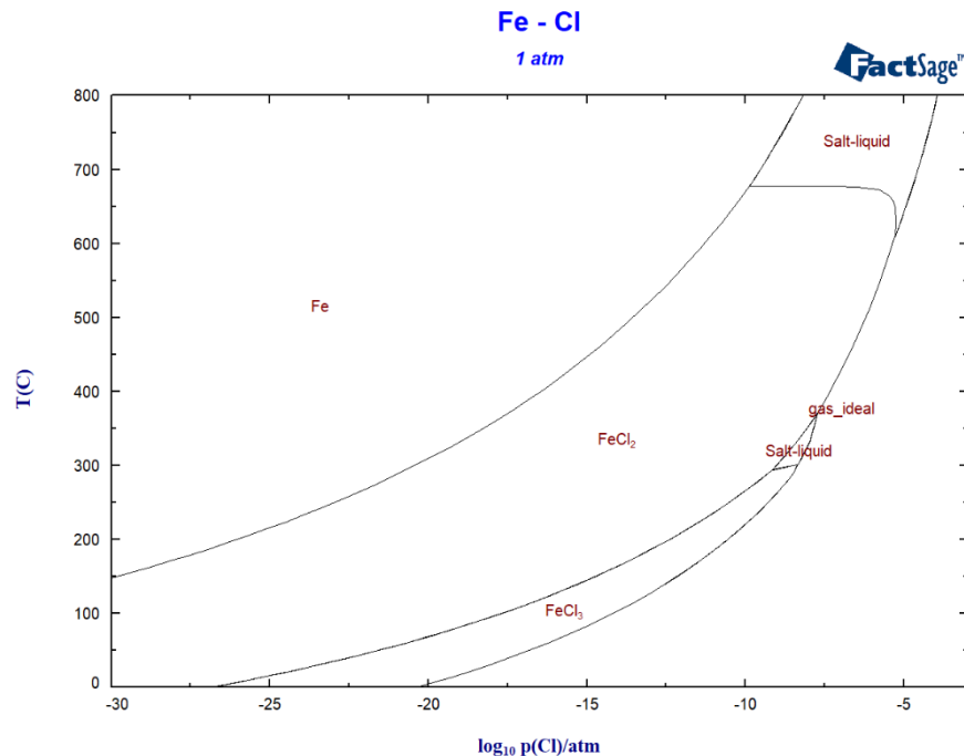
Abbildung 151: Fe-Cl Phasendiagramm mit \text{FeCl}_2 und \text{FeCl}_3 sowie Schmelzphase aus beidem in Abhängigkeit vom Chlorpartialdruck (Bale et al. 2016)
