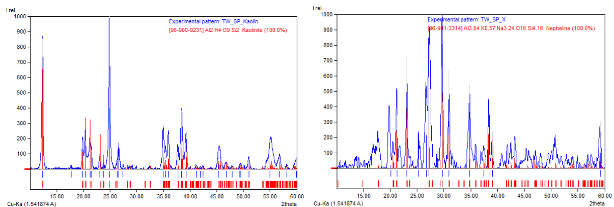
Abbildung 47: Pulverröntgendiffraktogramme in Reflexionsgeometrie mit Flächenprobenträger im Bragg-Brentano-Setup, 10-60° 2theta, (a) Kaolin unbehandelt, (b) Reaktionsprodukt Kaolin+NaCl (600°C, 24h, [N 2 , O 2 , H 2 O]), ausgewaschen und abfiltriert
