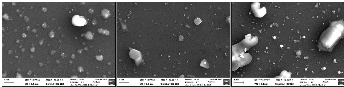
Abbildung 108: REM-Bilder Partikelprobe ohne Additiv, vor EÜ, 10s, Abströmseite, Temperaturreihe von 330°C, 380°C und 430°C als Substrattemperatur
