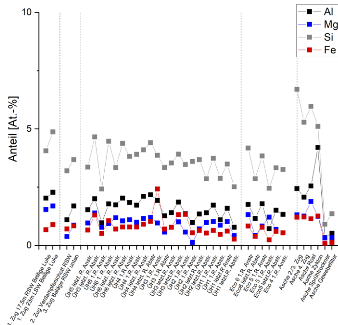
Abbildung 71: EDX-Belags- und Ascheanalysen GKS, Revision Oktober 2021, Aluminium, Magnesium Silizium und Eisen entlang der Anlage
