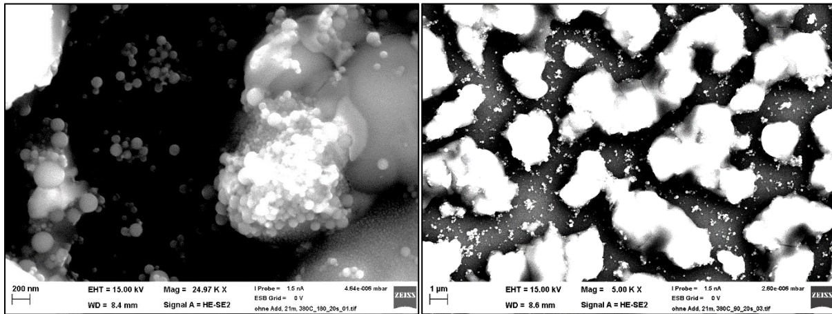
Abbildung 100: REM-Bild Partikelprobe ohne Additiv, nach EÜ, 380°C, 20s Detailaufnahme Anströmseite (a) und Übersicht Flanke 90° (b)
