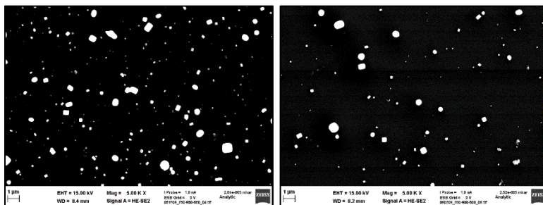
Abbildung 67: REM-Aufnahmen der abgeschiedenen NaCl-Partikel im Gastemperaturgradienten d) 750-650-500°C (Substrattemperatur 550°C) sowie e) 700-600-500°C (Substrattemperatur 500°C)
