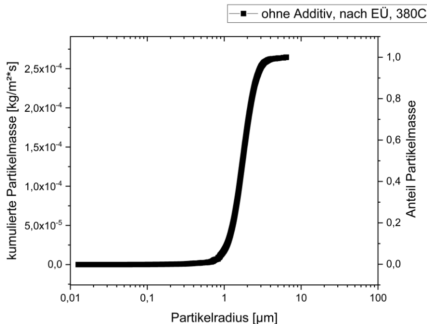
Abbildung 117: Partikelprobenahme MVV Gersthofen; kumulierte Partikelgrößenverteilung, Versuchstag ohne Additiv, Position nach Endüberhitzer, Sondentemperatur 380°C, Anströmseite, 10s im Rauchgas, ausgewertete Partikelzahl: 31.876
