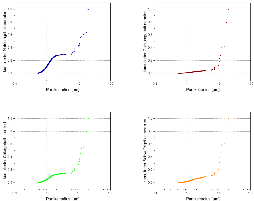
Abbildung 135: Partikelchemie der Elemente Natrium, Calcium, Chlor und Schwefel in Abhängigkeit von der Partikelgröße, MVV Gersthofen, mit Additiv, vor EÜ, Substrattemperatur 380°C, 10s im Rauchgas
