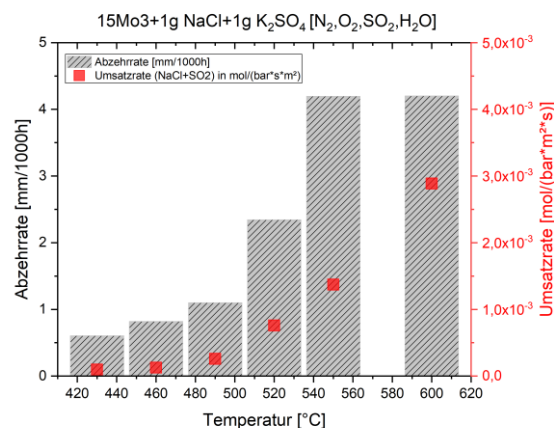
Abbildung 37: Laborexperimente Stahl+1g NaCl + 1g K 2 SO 4 , Umsatzrate (rot) und Korrosion (grau) als Temperaturreihe, in [N 2 , O 2 , H 2 O, SO 2 ], 4 Stunden
