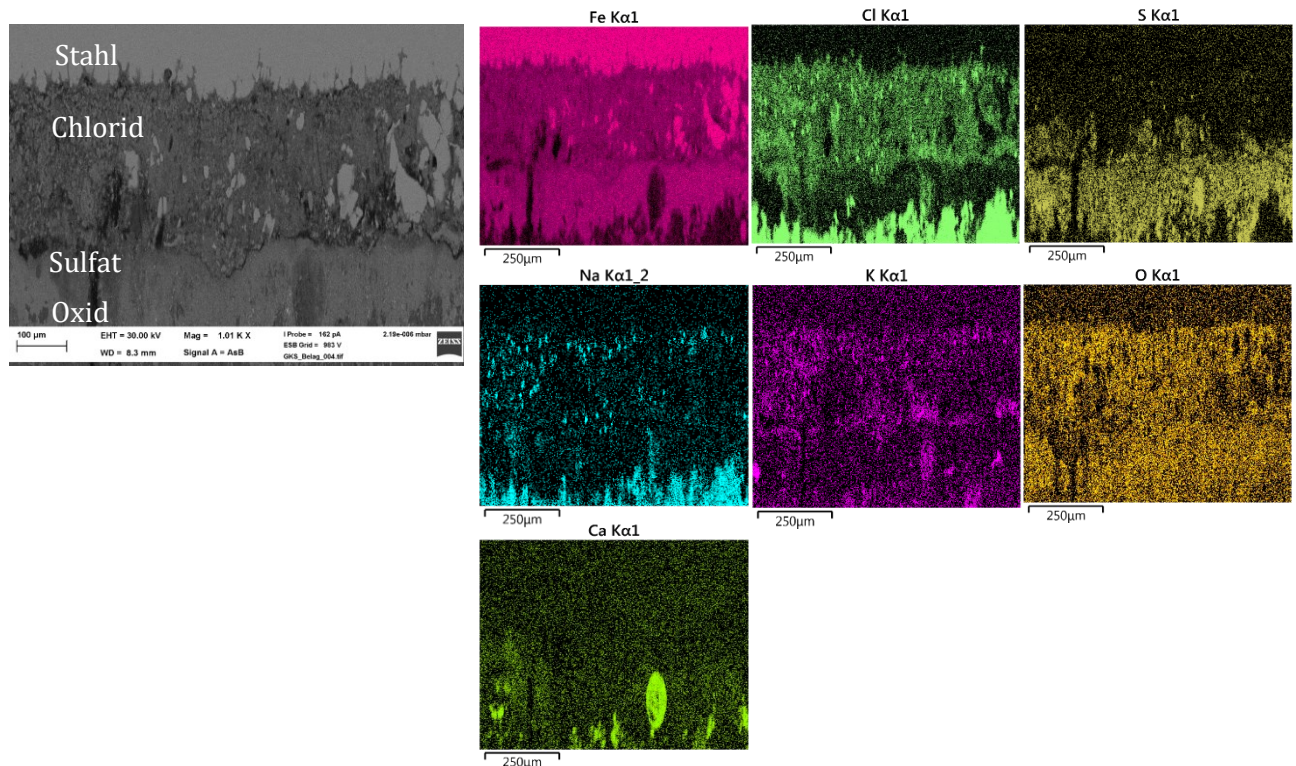
Abbildung 39: EDX-Mapping der Korrosionsschichten der Probe 15Mo3+1gNaCl+1g GKS-Belag, 600°C 4h, volle Atmosphäre
