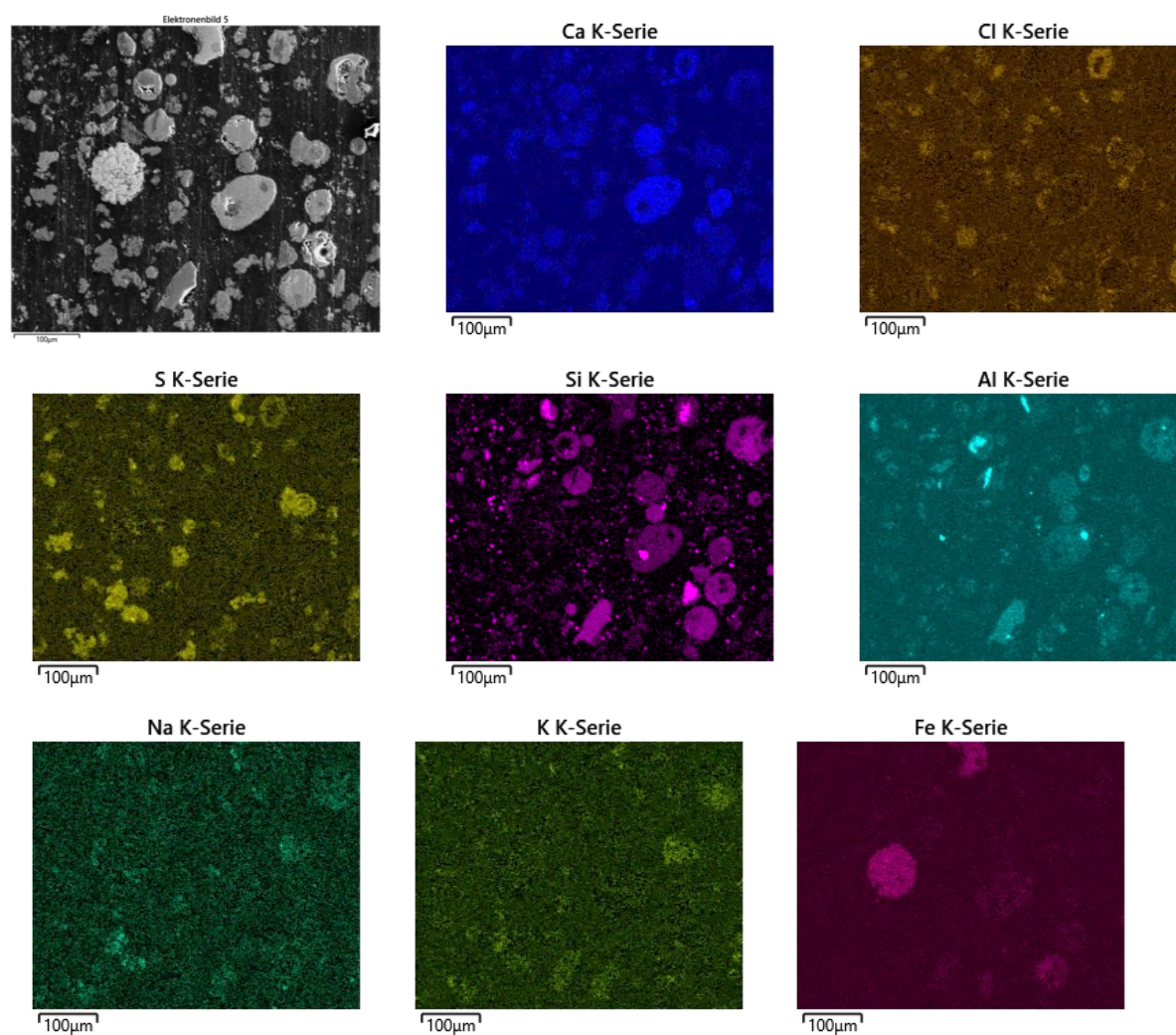
Abbildung 142: REM/EDX-Analysen Ascheprobe MVV Gersthofen, Trichter 2./3. Zug, Juli 2020
