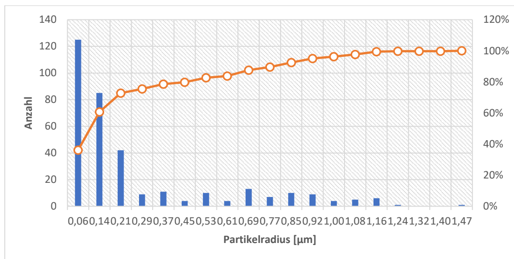
Abbildung 102: Partikelradius gegen Anzahl der Probe ohne Additiv, oberhalb EÜ, 380°C, 10s Anströmseite
