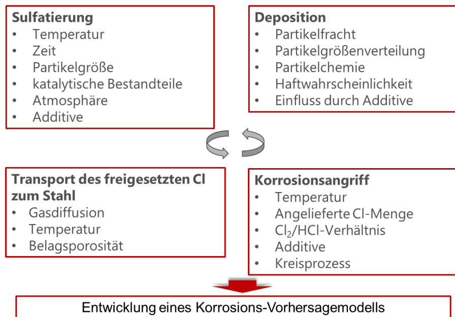
Abbildung 3: Modell-Parameter der Mechanismen zur Hochtemperatur-Chlorkorrosion
