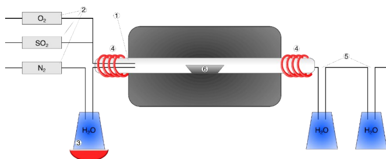
Abbildung 10: Schema des Versuchsaufbaus (1) Quarzrohr im Rohrofen, (2) Massendurchflussregler für Reaktionsgase, (3) beheizte Waschflasche für Wasserdampf in der Gasatmosphäre, (4) Heizmanschetten, (5) Waschflaschen zum Auffangen der Reaktionsgase
