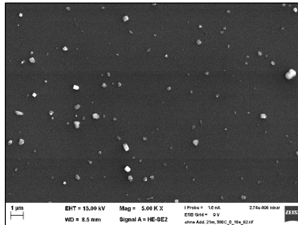
Abbildung 104: REM-Bilder Partikelprobe ohne Additiv, vor EÜ, 380°C, Abströmseite 10s im Rauchgasstrom
