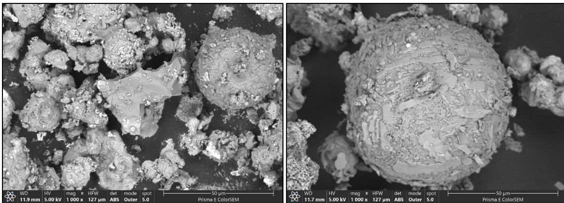
Abbildung 70: Detailaufnahme von Belagspartikeln, links: ÜH3 1. Reihe Anströmseite, rechts: ÜH6: 1. Reihe Anströmseite
