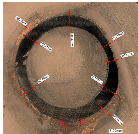
Abbildung 92: Digitalmikroskopie-Aufnahme des Querschnitts Austritt Überhitzer 2, MVV Gersthofen, Revision Oktober 2019, mit Restwand- und Belagsschichtdicken und Markierung des Analysebereichs für EDX (rotes Kästchen)
