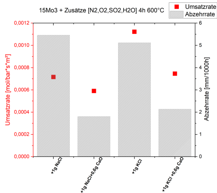
Abbildung 54: Umsatzrate und Abzehrrate der Laborexperimente Stahl+Salz mit und ohne Calciumoxidzugabe, 600°C, 4h
