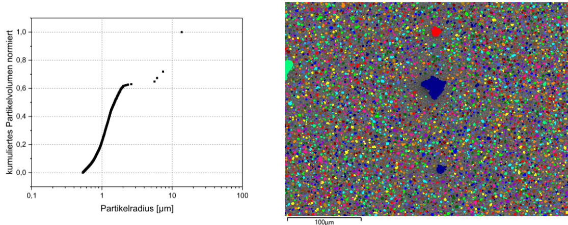
Abbildung 132: (a) kumuliertes Partikelvolumen (normiert) für einen Anteil der Partikel, MVV Gersthofen, ohne Additiv, vor EÜ, Substrattemperatur 380°C, 10s im Rauchgas, (b) Bildausschnitt für Partikelchemieauswertung, detektierte Partikelanzahl 6658
