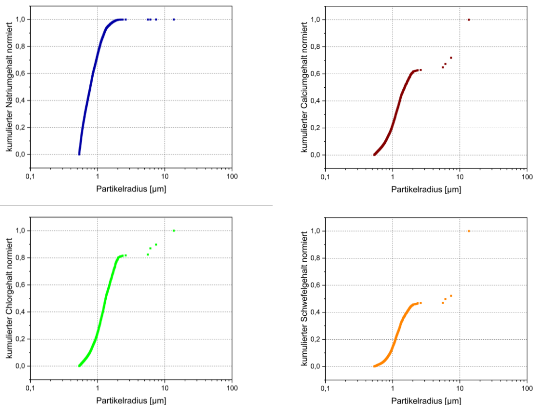
Abbildung 133: Partikelchemie der Elemente Natrium, Calcium, Chlor und Schwefel in Abhängigkeit von der Partikelgröße, MVV Gersthofen, ohne Additiv, vor EÜ, Substrattemperatur 380°C, 10s im Rauchgas
