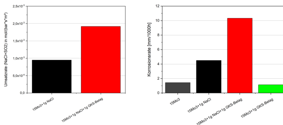
Abbildung 34: Laborexperimente Stahl+1g NaCl mit Anlagenbelag, Sulfatierungsrate (a) und Korrosionsrate (b) bei 600°C, 4 Stunden, Atmosphäre [N 2 , O 2 , H 2 O, SO 2 ]
