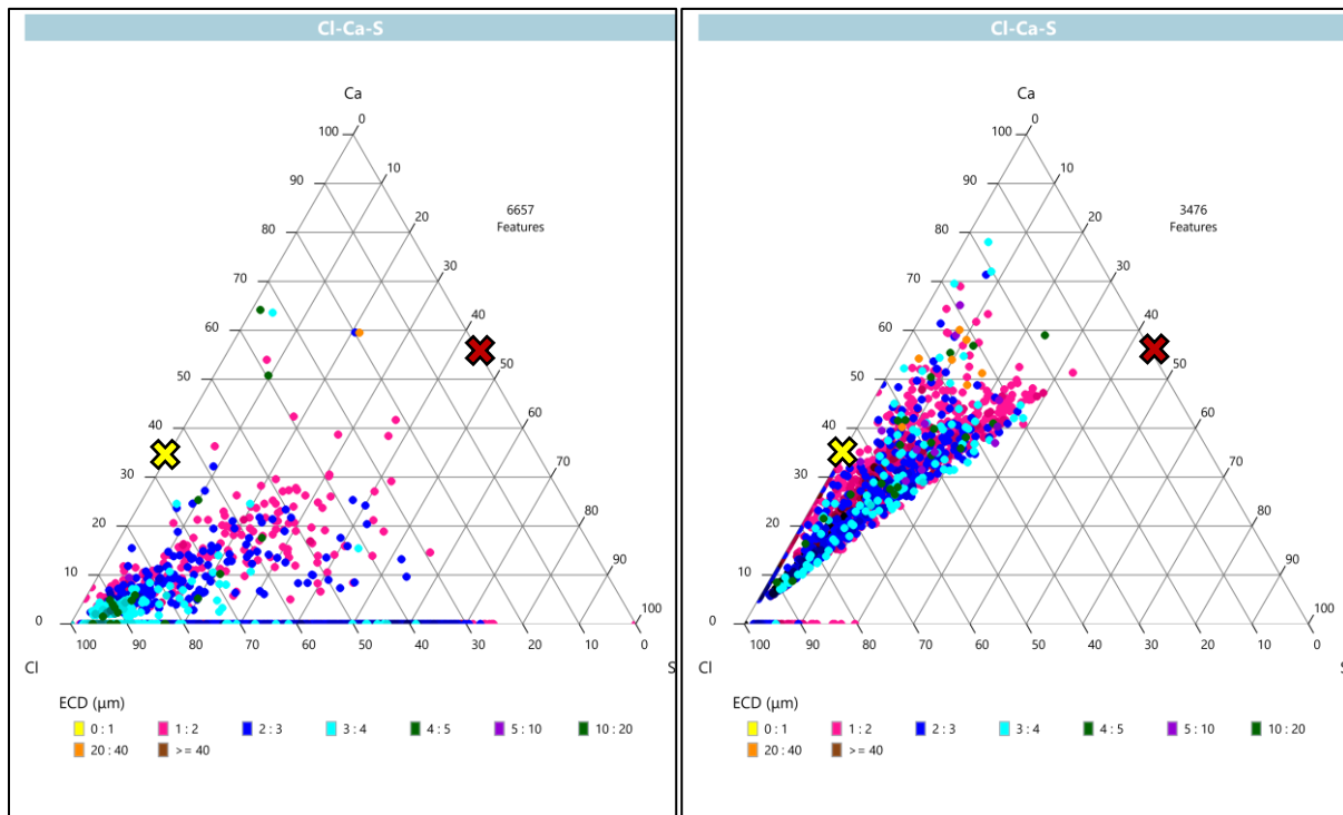
Abbildung 137: ternäre Korrelation der Elemente Calcium mit Chlor und Schwefel, (a) ohne Additiv, (b) mit Additiv, MVV Gersthofen, vor EÜ, Substrattemperatur 380°C, 10s im Rauchgas, Farbkodierung entspricht dem Partikeldurchmesser (equivalent circular diameter ECD), normierte EDX-Daten in Gew.-%, gelbes Kreuz: Stöchiometrie \text{CaCl}_2 , rotes Kreuz: \text{CaSO}_4
