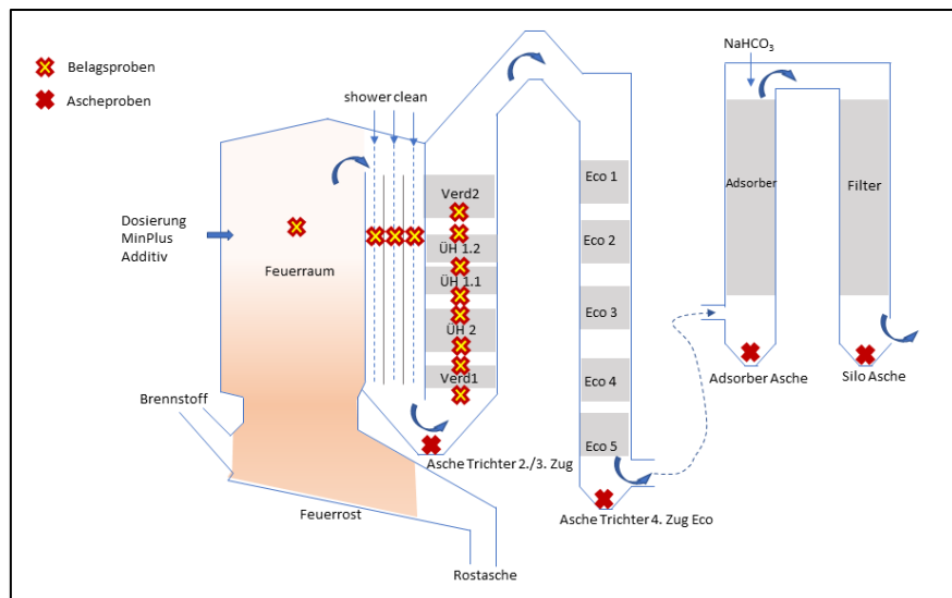
Abbildung 19: Skizze der Anlage MVV Gersthofen, Aschenahme- und Belagsproben-Positionen, (nach (Biermann and Mani 2022))
