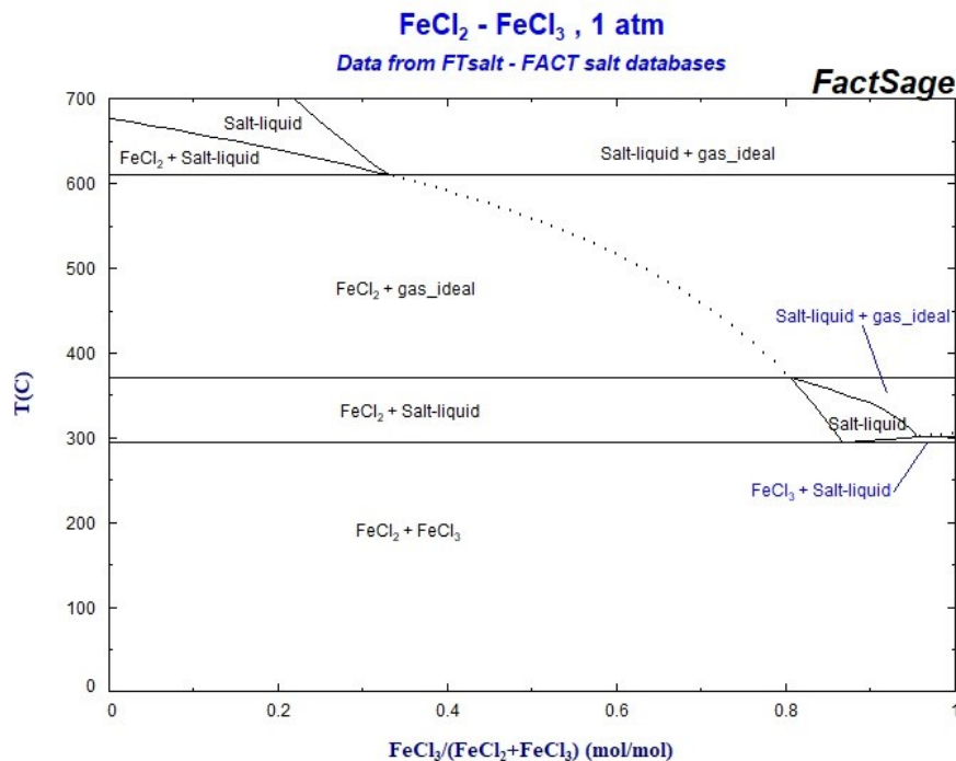
Abbildung 152: Phasendiagramm \text{FeCl}_2 und \text{FeCl}_3 (Bale et al. 2016)
