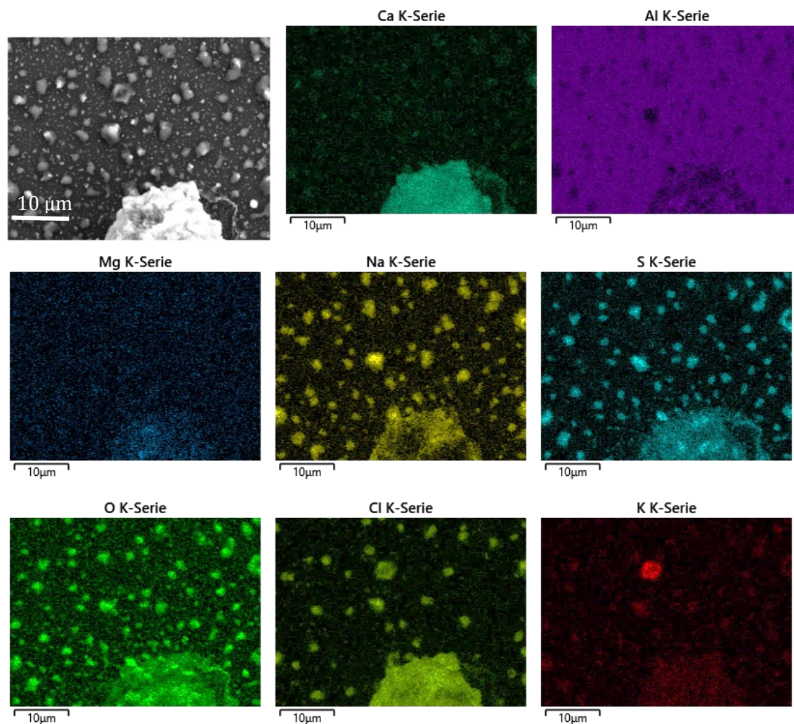
Abbildung 122: REM- (SE-Detektor) und EDX-Mappings der Probe mit Additiv, nach EÜ, 430°C, Anströmseite, 10s, 2.500-fache Vergrößerung
