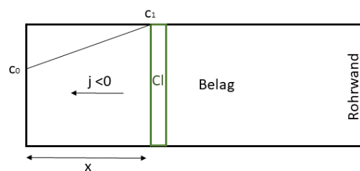
Abbildung 149: Skizze: Diffusion von freigesetztem Chlor in Belagstiefe x durch den Belag mit Konzentrationsüberhöhung c_1 im Vergleich zu äußerem Chlorgehalt c_0
