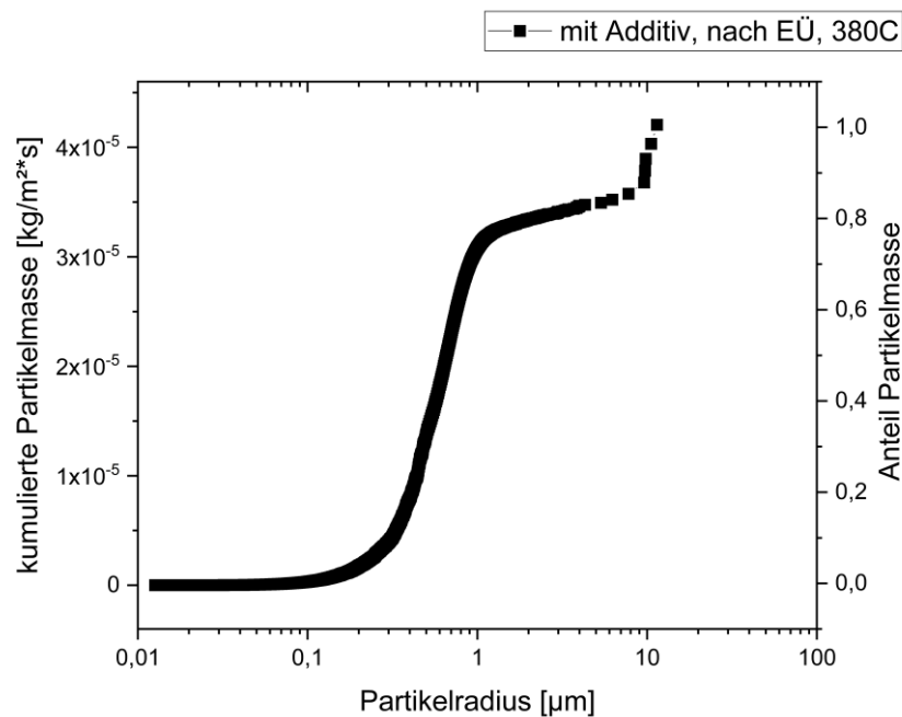
Abbildung 119: Partikelprobenahme MVV Gersthofen; kumulierte Partikelgrößenverteilung, Versuchstag mit Additiv, Position nach Endüberhitzer, Sondentemperatur 380°C, Anströmseite, 10s im Rauchgas, ausgewertete Partikelzahl: 57.067
