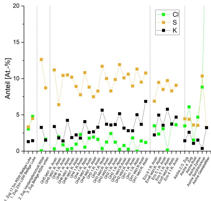
Abbildung 74: EDX-Belags- und Ascheanalysen GKS, Revision Oktober 2021, Schwefel und Chlor mit jeweils Calcium, Natrium oder Kalium
