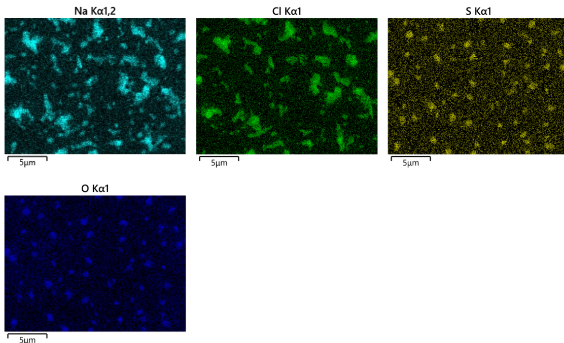
Abbildung 64: EDX-Mapping der Partikel aus Abbildung 63 b) nach 4 Minuten im Gasstrom mit Sauerstoff (6 vol.-%) und \text{SO}_3 (100 ppmv, aus Ammoniumsulfat), bei 600^\circ\text{C}
