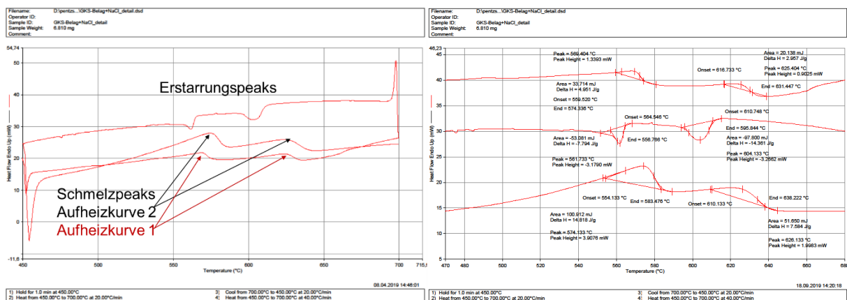
Abbildung 41: DSC-Messungen des Gemisches NaCl+Anlagenbelag (Massenverhältnis 1:1), gesamter Temperaturbereich von 400°C-700°C (a), Auswertung der Peaks: 1. Aufheizen oben, Abkühlen mitte, 2. Aufheizen unten (b)
