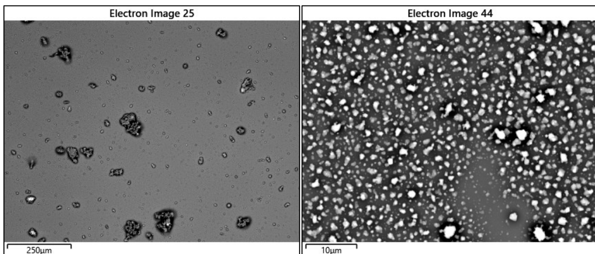
Abbildung 146: REM-Aufnahmen: Partikelproben MHKW Rosenheim, mit Additiv, nach EÜ, Anströmseite, Substrattemperatur 380°C, 10s im Rauchgas
