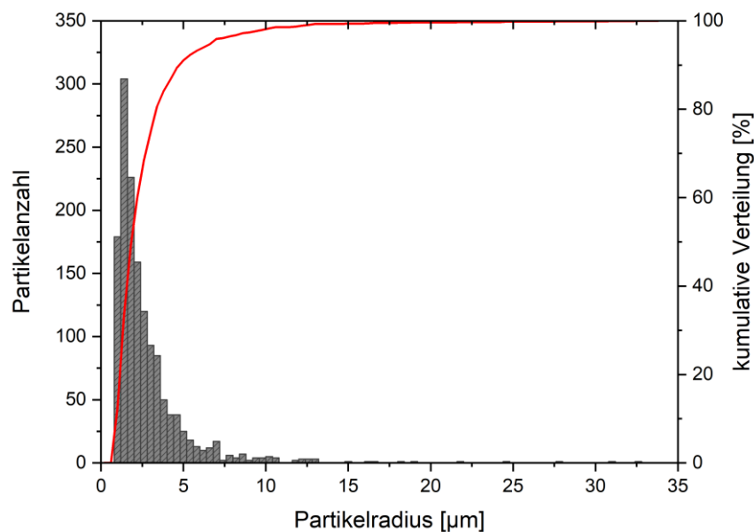
Abbildung 56: Partikelradius-Größenverteilung des MinPlus-Additivs, bestimmt via REM mittels fein verteiltem Pulver auf Si-Plättchen, 1450 Partikel
