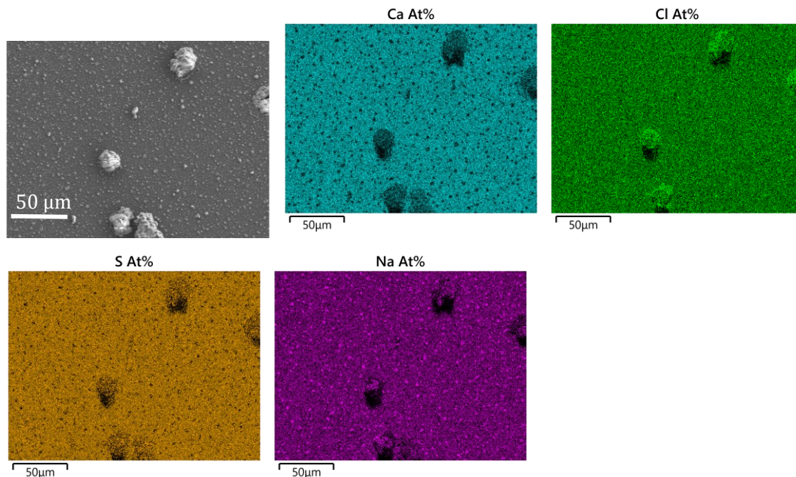
Abbildung 123: REM (SE-Detektor) und EDX-Mappings der Probe mit Additiv, vor EÜ, 330°C, Anströmseite, 10s, 500-fache Vergrößerung
