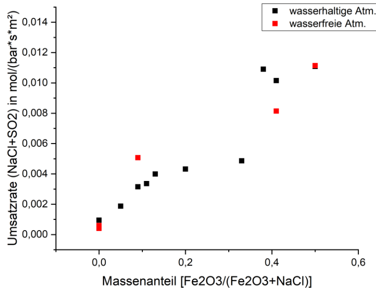
Abbildung 31: Umsatzrate bei Variation des Massenanteils an Eisenoxid als Reaktionszusatz, Stahl+NaCl, 600°C
