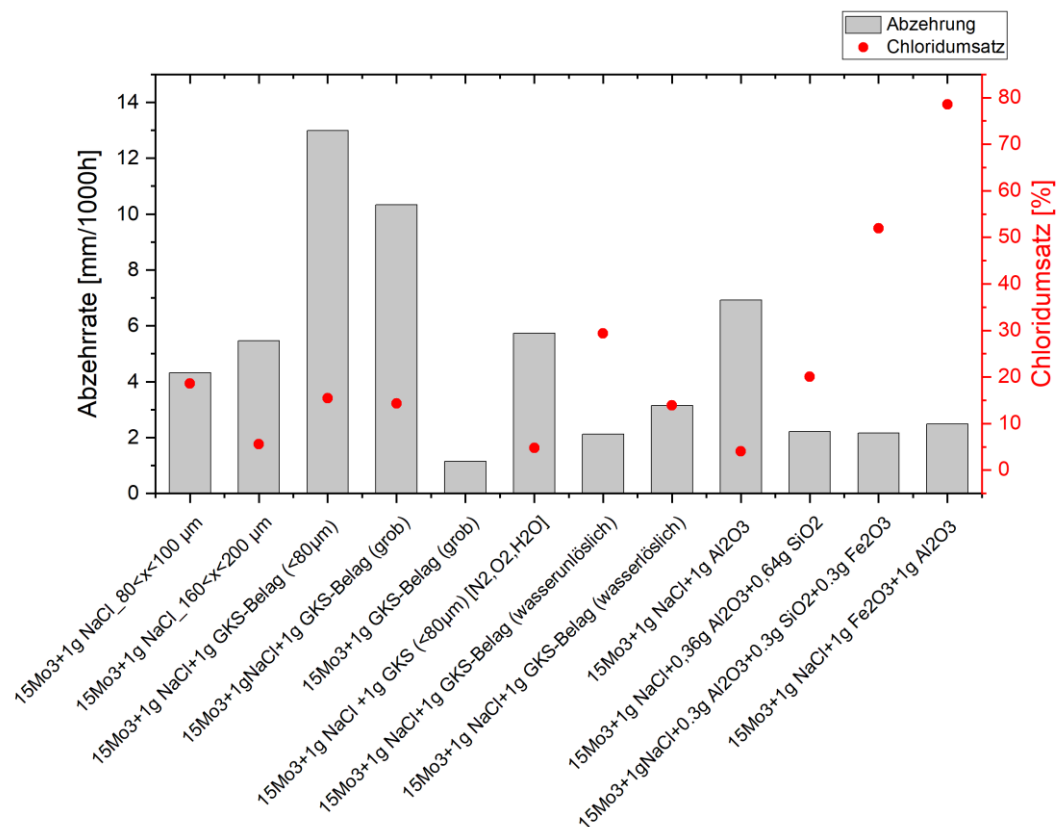
Abbildung 35: Laborexperimente: Stahl+NaCl mit Zusätzen von GKS-Belag und unterschiedlichen Oxiden, Umsatz in [%] (rot) und Korrosion [mm/1000h] (grau) bei 600°C, 4 Stunden, [N 2 , O 2 , H 2 O, SO 2 ]
