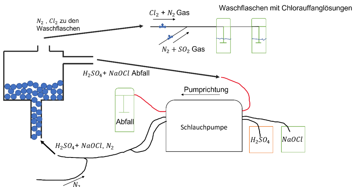
Abbildung 13: schematische Darstellung des Aufbaus zur Fließgleichgewichtserzeugung von \text{Cl}_2 (Krupkov 2022)
