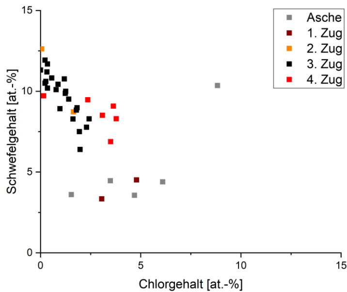
Abbildung 77: EDX-Belags- und Ascheanalysen GKS, Revision Oktober 2021, Auftragung Schwefel gegen Chlor, Messpositionen entlang der gesamten Anlage (ohne Asche Gewebefilter: Cl=33 At.-%)
