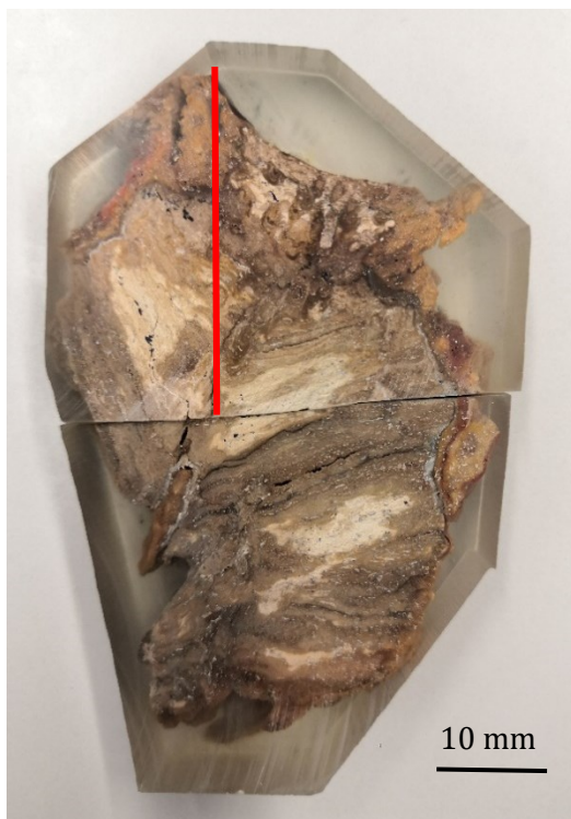
Abbildung 94: Belagsbart MVV Gersthofen, Überhitzer 2 Anströmseite, Oktober 2019, mit eingezeichnetem REM/EDX Scan (rote Linie)
