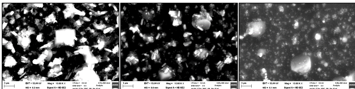
Abbildung 109: REM-Bilder Partikelprobe mit Additiv, vor EÜ, 10s, Anströmseite, Temperaturreihe von 330°C, 380°C und 430°C als Substrattemperatur
