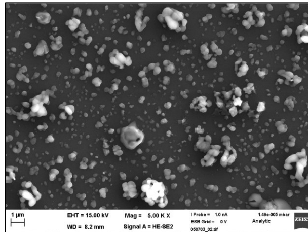
Abbildung 65: Agglomeratbildung von kubischen Salzpartikeln bei Reaktion mit Schwefeldioxid, 1 Minute im Gasstrom mit Sauerstoff (6 vol.-%) und Schwefeldioxid (0,7 vol.%) sowie anteilig \text{SO}_3 durch Eisenoxidkatalysator, Temperaturgradient 750-650-550°C
