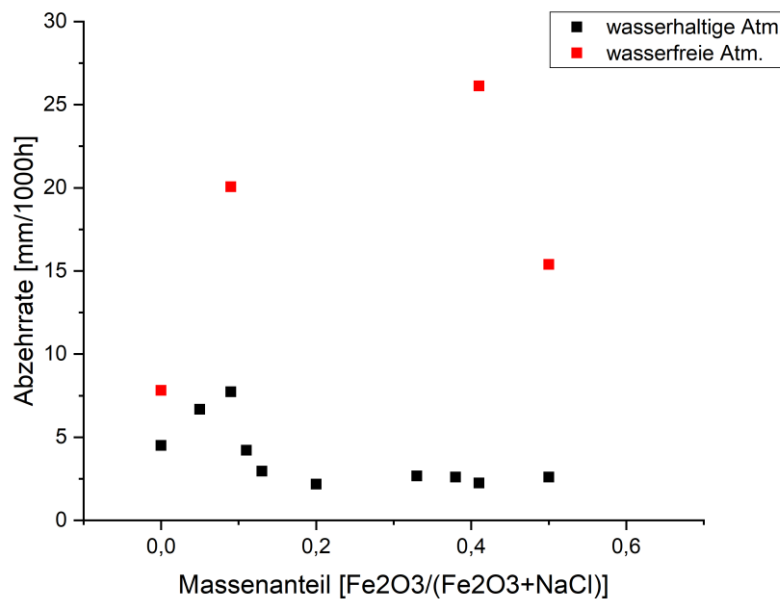
Abbildung 32: Abzehrung bei Variation des Massenanteils an Eisenoxid als Reaktionszusatz, Stahl+NaCl, 600°C
