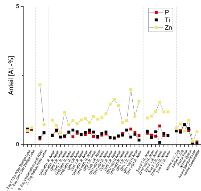
Abbildung 75: EDX-Belags- und Ascheanalysen GKS, Revision Oktober 2021, Phosphor, Titan und Zink entlang der Anlage
