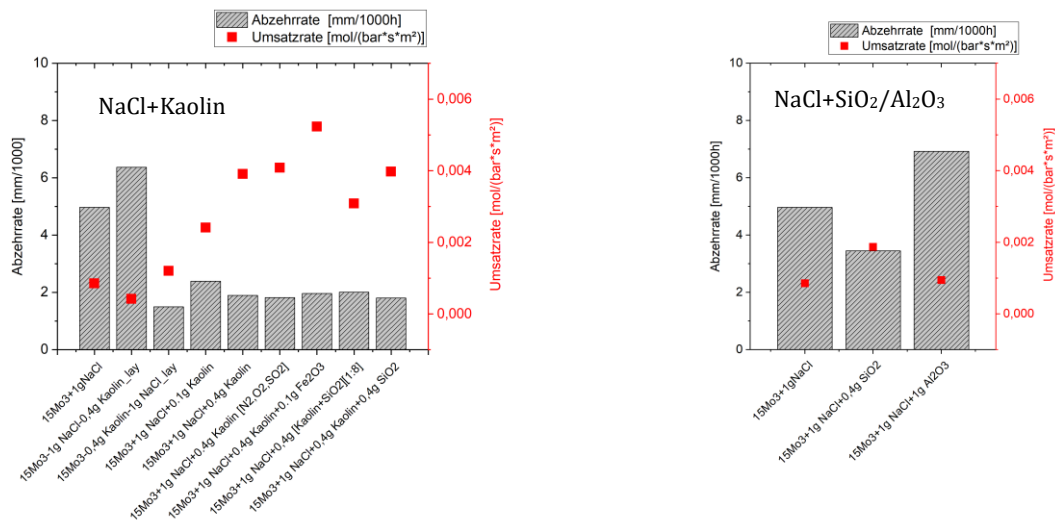
Abbildung 48: Laborexperimente mit Stahl+NaCl und Zugabe von Kaolin bei 600°C für 4h, [\text{N}_2, \text{O}_2, \text{H}_2\text{O}, \text{SO}_2] (wenn nicht anders angegeben)
