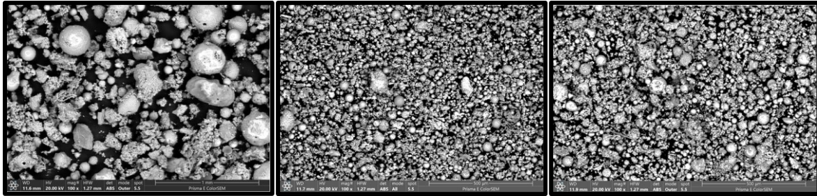
Abbildung 69: REM-Aufnahmen links: Asche 2./3. Zug, mitte: Belag ÜH6 letztes Rohr Abströmseite, rechts: Belag ÜH4 1. Rohr Anströmseite
