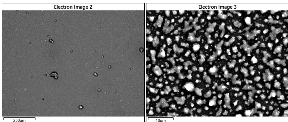
Abbildung 114: Partikelprobenahme MVV Gersthofen; REM-Aufnahme, ohne Additiv, Position vor Endüberhitzer, Substrattemperatur 380°C, Anströmseite, 10s im Rauchgas, niedrige und hohe Vergrößerung
