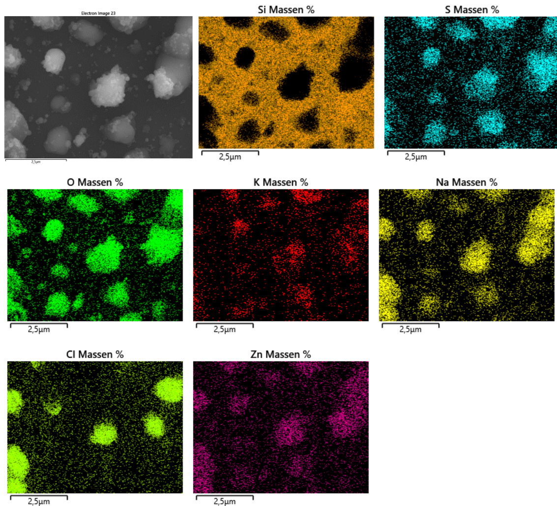
Abbildung 121: REM- und EDX-Mappings der Probe ohne Additiv, nach EÜ, 430°C, Anströmseite, 10s, 10.000-fache Vergrößerung
