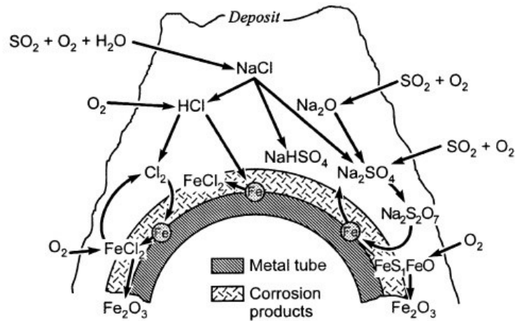
Abbildung 7: Reaktionsschema der chlorinduzierten Korrosion durch Sulfatierung der Alkalichloride im Belag (Nielsen et al. 2000)
