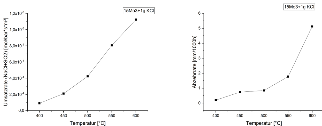
Abbildung 24: Temperaturreihe für die Umsatzrate (a) und Abzehrung (b) von 15Mo3 mit 1g KCl unter voller Atmosphäre
