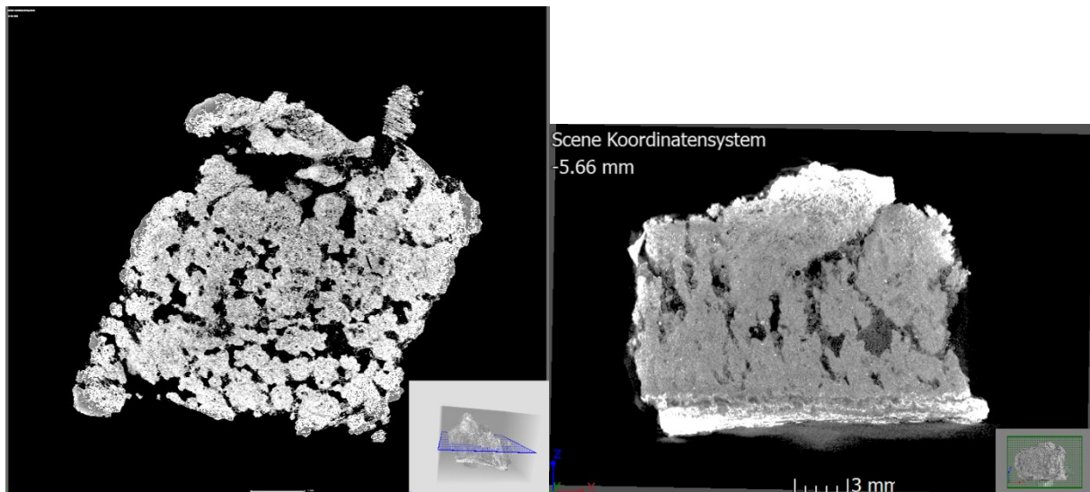
Abbildung 5: Computertomographie-Scan durch einen Anlagenbelag; a) Querschnitt b) Frontansicht, unten rohnahe Bereich, oben Belagsaußenseite (Ott 2017)
