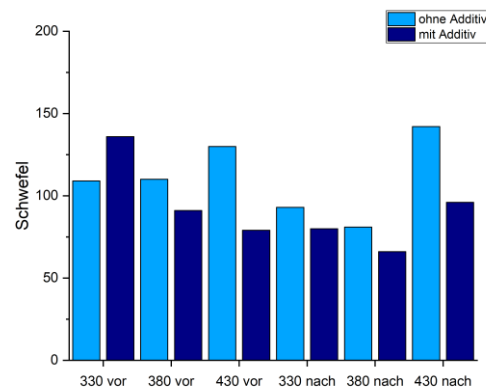
Abbildung 131: EDX Signalintensitäten für Chlor und Schwefel, vor und nach EÜ, ohne und mit Additiv für die unterschiedlichen Substrattemperaturen 330°C, 380°C, 430°C
