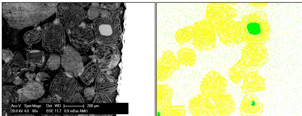
Abbildung 27: (a) stufenweise Sulfatierung kubischer NaCl-Partikel zu Sulfaten, (b) EDX-Mapping mit Schwefel (gelb) und Chlor (grün) (Ott 2017)
