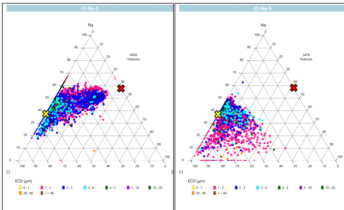
Abbildung 136: ternäre Korrelation der Elemente Natrium mit Chlor und Schwefel, (a) ohne Additiv (6658 analysierte Partikel), (b) mit Additiv (3476 analysierte Partikel); MVV Gersthofen, vor EÜ, Substrattemperatur 380°C, 10s im Rauchgas, Farbkodierung entspricht dem Partikeldurchmesser (equivalent circular diameter ECD), normierte EDX-Daten in Gew.-%, gelbes Kreuz: Stöchiometrie NaCl, rotes Kreuz: \text{Na}_2\text{SO}_4
