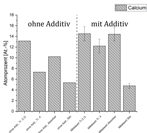
Abbildung 140: Calciumgehalte in den Aschen: Trichter 2./3. Zug, 4. Zug, Absorber und Silo, ohne Additiv Jan22 und mit Additiv Mittelwert aus Jan22, Okt21
