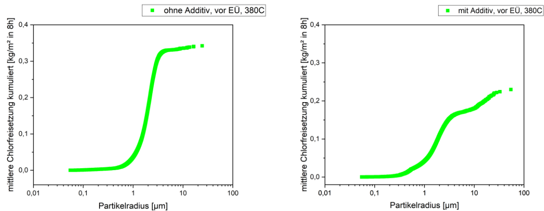
Abbildung 139: mittlere Chlorfreisetzung kumuliert aus m_{\text{Cl}}^{\text{frei}}(t) , nach 8h, ohne und mit Additivedosierung, MVV Gersthofen, vor Endüberhitzer, Substrattemperatur 380^\circ\text{C} , 10s im Rauchgas
