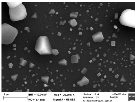
Abbildung 59: deponierte NaCl-Partikel nach einer Minute im Gasstrom aus Sauerstoff (6 vol.-%) und Schwefeldioxid (0,7 vol.%) bei 600°C
