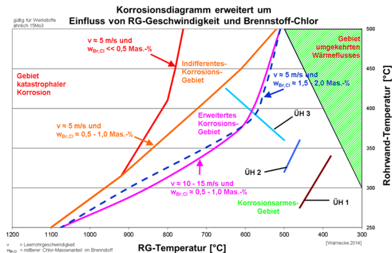
Abbildung 2: Flingernsches Korrosionsdiagramm mit Erweiterungen aus Daten des Gemeinschaftskraftwerk Schweinfurt, korrosive Bereiche von Berührungsheizflächen in Abfallverbrennungsanlagen, Berücksichtigung der Rauchgasgeschwindigkeit, des Chlorgehalts und der eingesetzten Werkstoffe, Chlorgehalt in Gew.-% (wasserfrei), Strömungsgeschwindigkeit als lokale Normalgeschwindigkeit (in Betriebszustand), Asche- und Wassergehalt des Brennstoffs ~25 Gew.-%, O 2 ~ 8 Vol.-%, (Warnecke 2014)
