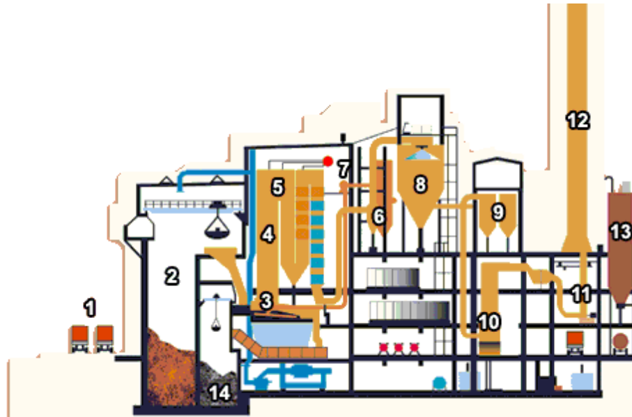
Abbildung 1: schematischer Aufbau einer Müllverbrennungsanlage, mit 1 Müllanlieferung, 2 Müllbunker, 3 Verbrennungsrost, 4 SNCR-Entstickung, 5 vier-zügiger Kessel, 6 Multizyklon, 7 Rauchgasrückführung, 8 Sprühtrockner, 9 Gewebefilter, 10 zweistufiger Wäscher, 11 Saugzug, 12 Kamin, 13 Reststoffsilos, 14 Schlackebunker (nach (GKS Schweinfurt 2022))
