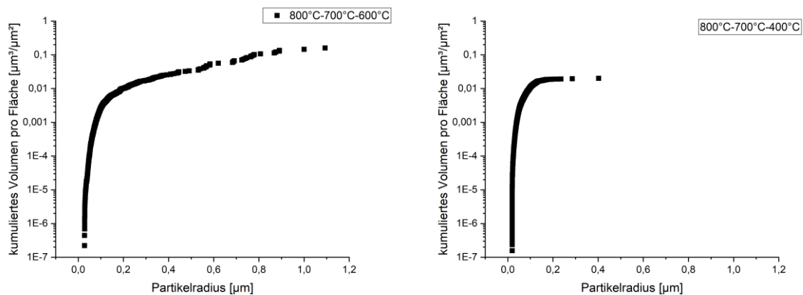
Abbildung 68: kumulierte Partikelvolumenverteilung für die Temperaturgradienten von a) 800-700-600°C und b) 800-700-400°C
