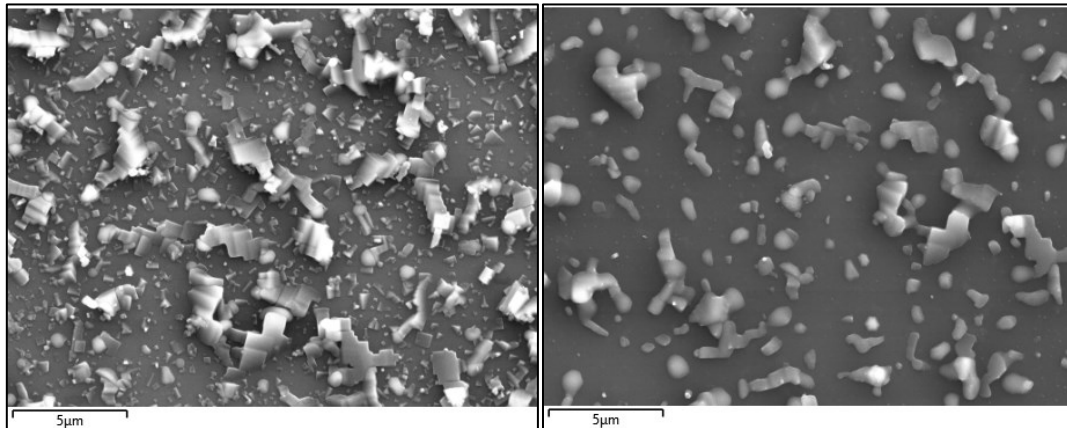
Abbildung 63: REM-Aufnahmen a) Abscheidung NaCl-Partikel unter N_2 mittels Zerstäuber auf Si-Substrat bei 600^\circ\text{C} ; b) Partikel nach 4 Minuten im Gasstrom mit Sauerstoff (6 vol.-%) und \text{SO}_3 (100 ppmv, aus Ammoniumsulfat), bei 600^\circ\text{C}
