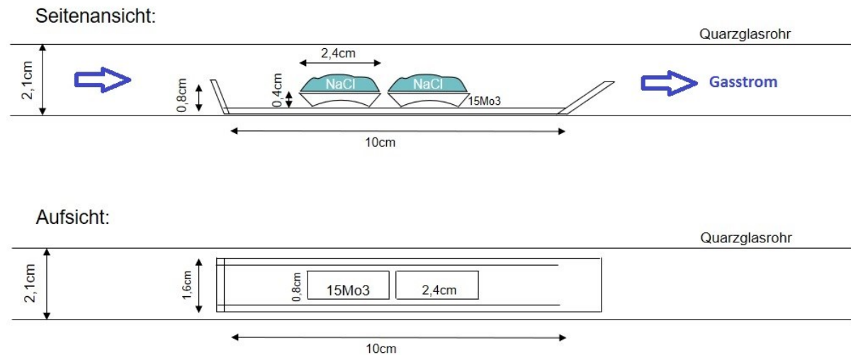
Abbildung 11: Probenanordnung einer 15Mo3+NaCl-Probe im Quarzrohr (Ott 2017)
