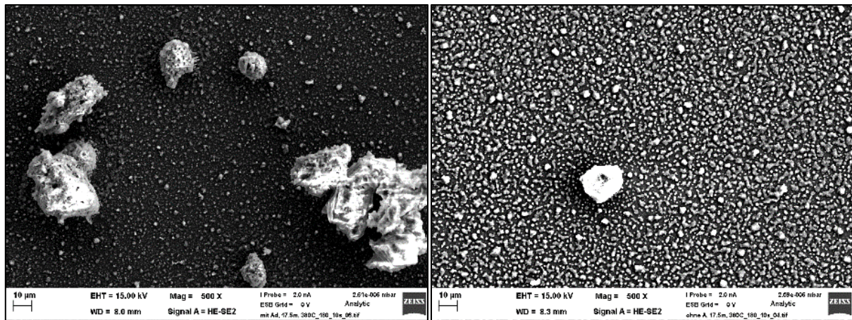
Abbildung 111: Vergleich der REM-Bilder mit Additiv (a) und ohne Additiv (b) für die Probenposition vor EÜ, 10s, Anströmseite, Übersichtsaufnahme 500x
