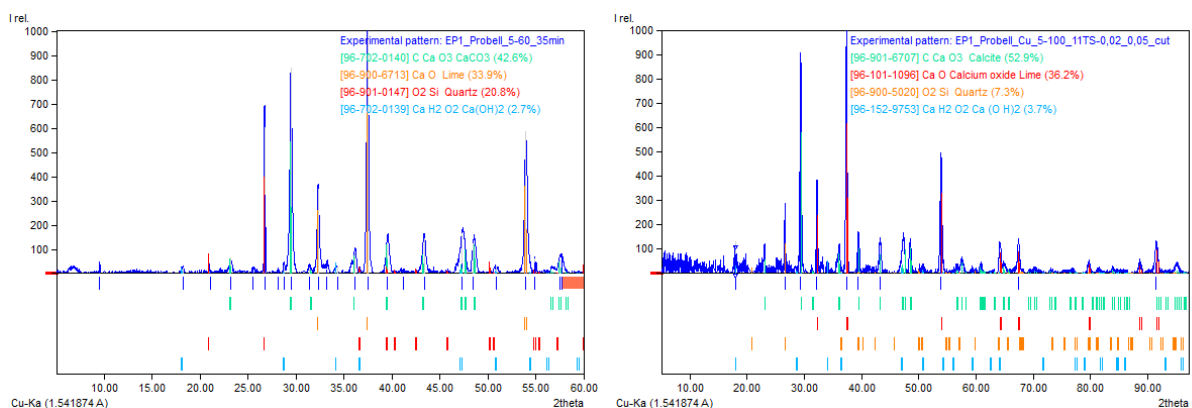
Abbildung 57: Pulverröntgendiffraktogramme MinPlus-Additiv unbehandelt, (a) in Reflexionsgeometrie mit Flächenprobenträger im Bragg-Brentano-Setup, 5-60° 2theta, (b) in Transmissionsgeometrie mit Glaskapillare im Debye-Scherrer-Setup, 5-100° 2theta, Quantifizierung von \text{CaCO}_3 , \text{CaO} , \text{CaOH} und \text{SiO}_2
