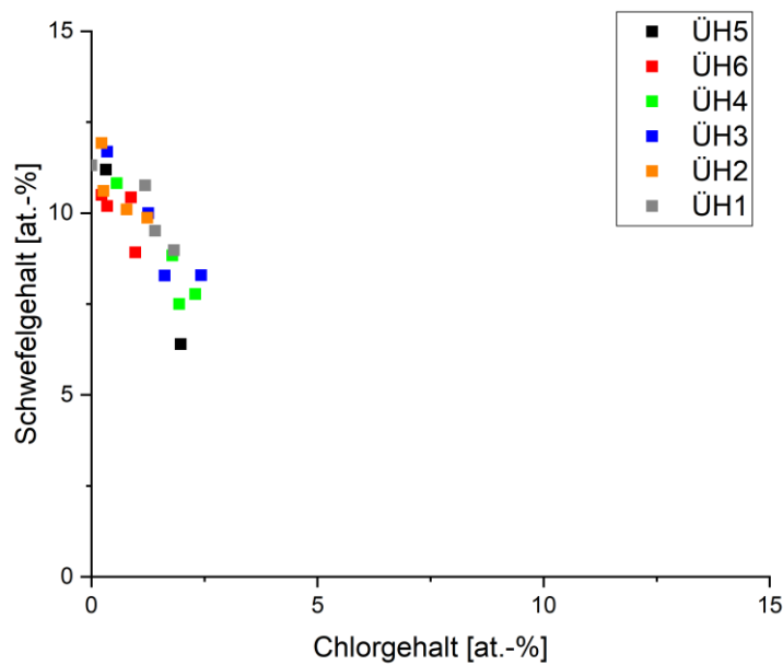
Abbildung 78: EDX Belags- und Ascheanalysen GKS, Revision Oktober 2021, Auftragung Schwefel gegen Chlor, Messpositionen im 3. Zug
