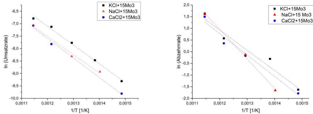
Abbildung 25: Arrheniusauftrag für die Umsatzrate (a) und Abzehrung (b) von 15Mo3 mit 1g KCl unter voller Atmosphäre
