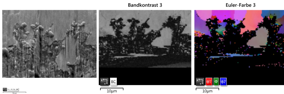
Abbildung 40: EBSD-Aufnahme der Grenzschicht zwischen Eisenchloridschicht und Stahl für die Probe 15Mo3+1gNaCl+1gGKS-Belag, 600°C, 4h, volle Atmosphäre, REM-Bild (a), Bandkontrast (b), Darstellung in Eulerfarben (c)
