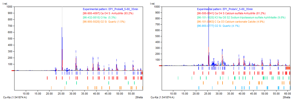
Abbildung 96: Pulverröntgendiffraktogramme in Reflexionsgeometrie mit Flächenprobenträger im Bragg-Brentano-Setup, 5-60° 2theta, (a) Anlage MVV Gersthofen (b) Anlage Gemeinschaftskraftwerk Schweinfurt GKS
