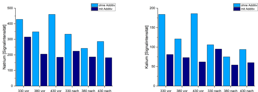
Abbildung 129: EDX-Signalintensitäten für Natrium und Kalium, vor und nach EÜ, ohne und mit Additiv für die unterschiedlichen Substrattemperaturen 330°C, 380°C, 430°C
