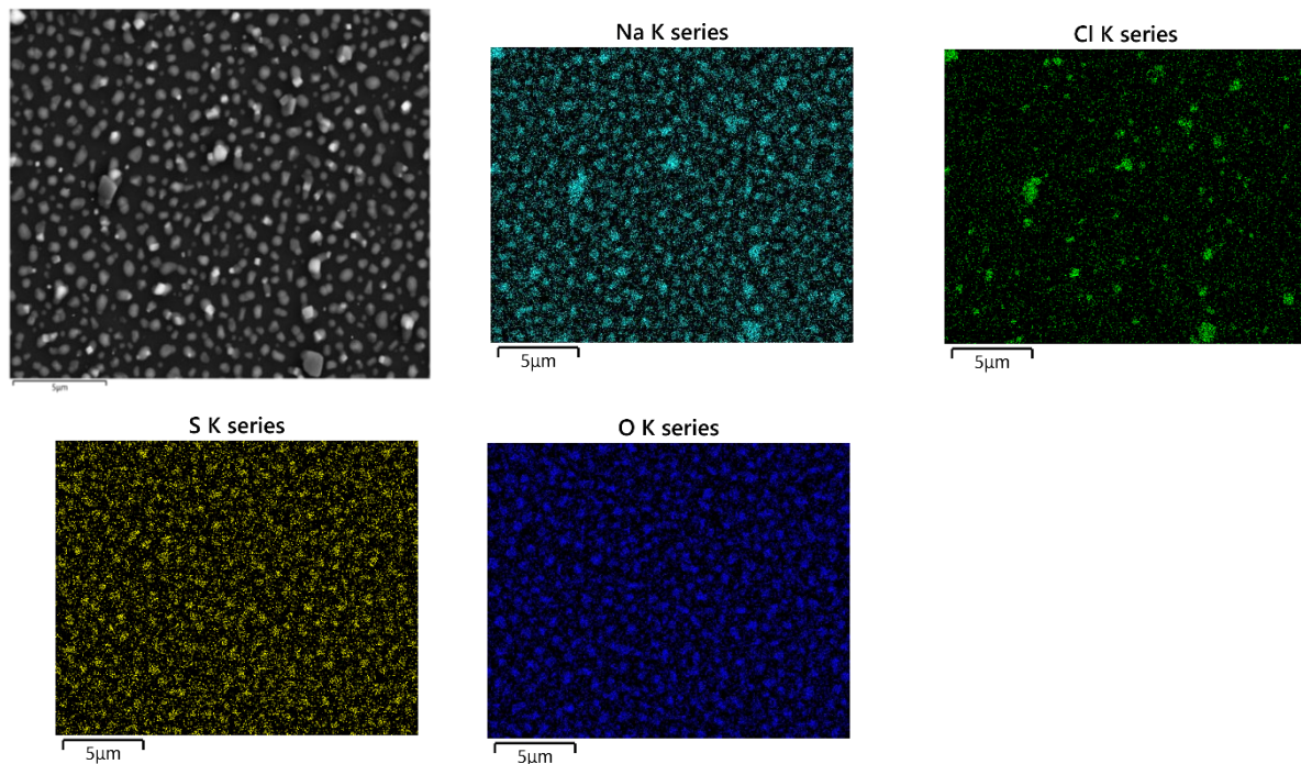
Abbildung 60: deponierte NaCl-Partikel nach fünf Minuten im Gasstrom aus Sauerstoff (6 vol.-%) und Schwefeldioxid (0,7 vol.%) bei 600°C
