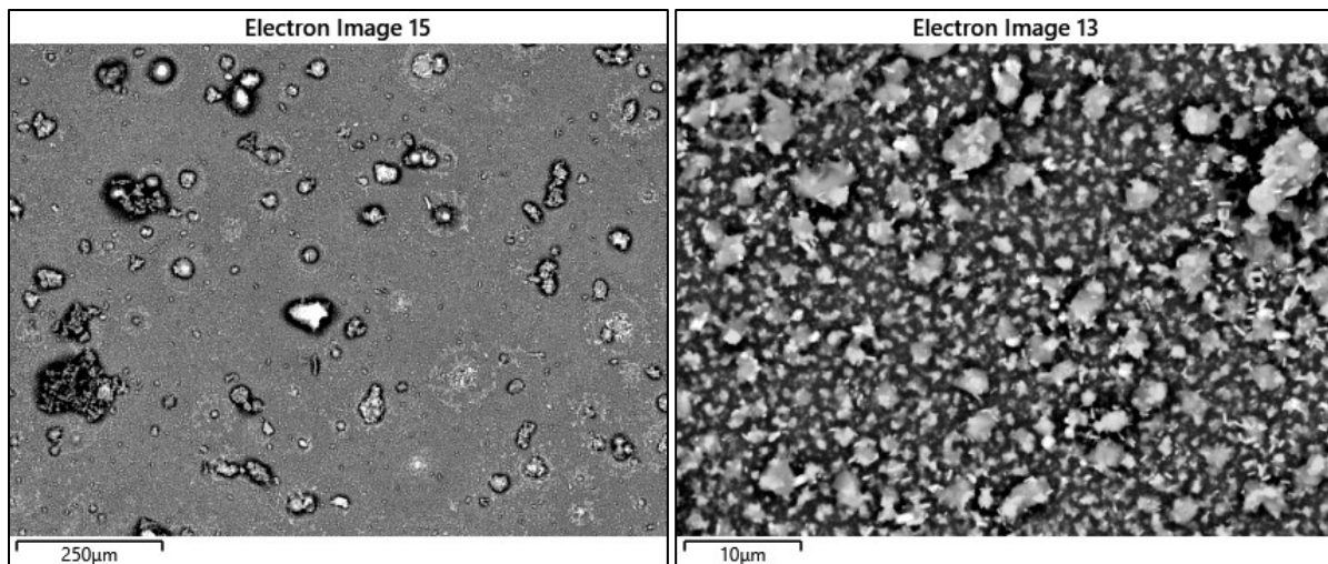
Abbildung 116: Partikelprobenahme MVV Gersthofen; REM-Aufnahmen, Versuchstag mit Additiv, Position vor Endüberhitzer, Sondentemperatur 380°C, Anströmseite, 10s im Rauchgas, niedrige und hohe Vergrößerung
