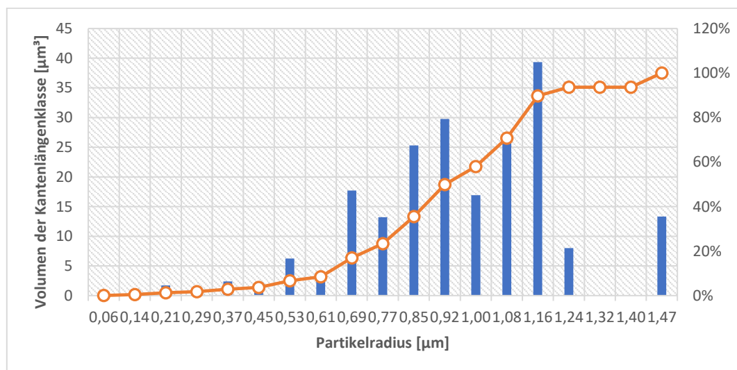
Abbildung 103: Partikelradius gegen Volumen der Kantenlängenklasse für die Probe ohne Additiv, oberhalb EÜ, 380°C, 10s Anströmseite
