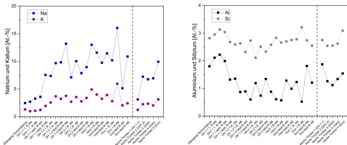
Abbildung 90: EDX-Belags- und Ascheanalysen MHKW Rosenheim, Probenahme Mai 2022 (mit MinPlus-Additiv), Calcium, Chlor, Schwefel, Natrium und Kalium sowie Aluminium und Silizium (andere y-Achsenskalisierung) entlang der Anlage
