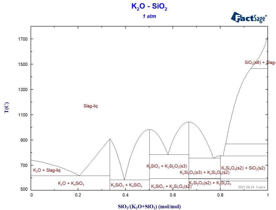
Abbildung 8: binäres Phasendiagramm \text{SiO}_2\text{-K}_2\text{O} (berechnet mit FactSage nach (Bale et al. 2016))
