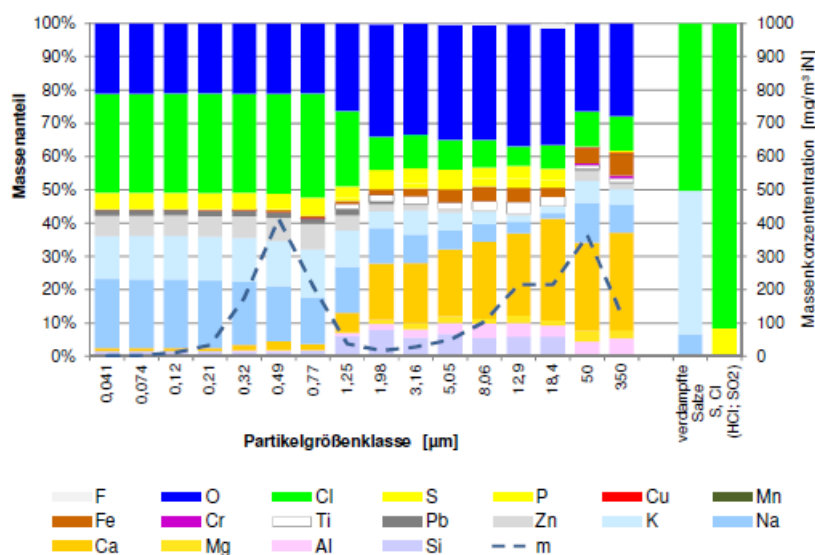
Abbildung 4: Partikelgrößenverteilung sowie -chemie, gemessen im 3. Zug des Gemeinschaftskraftwerks Schweinfurt im Rahmen des VoKos-Projekts (Warnecke et al. 2018)
