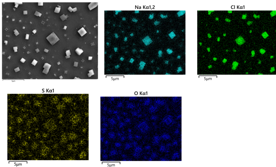
Abbildung 62: Sulfatierung von NaCl-Partikeln nach 1,5 Minuten im Gasstrom aus Sauerstoff (2 vol.-%) und Schwefeldioxid (0,7 vol.%), sowie anteilig \text{SO}_3 durch Eisenoxiddkatalysator, bei 600^\circ\text{C}
