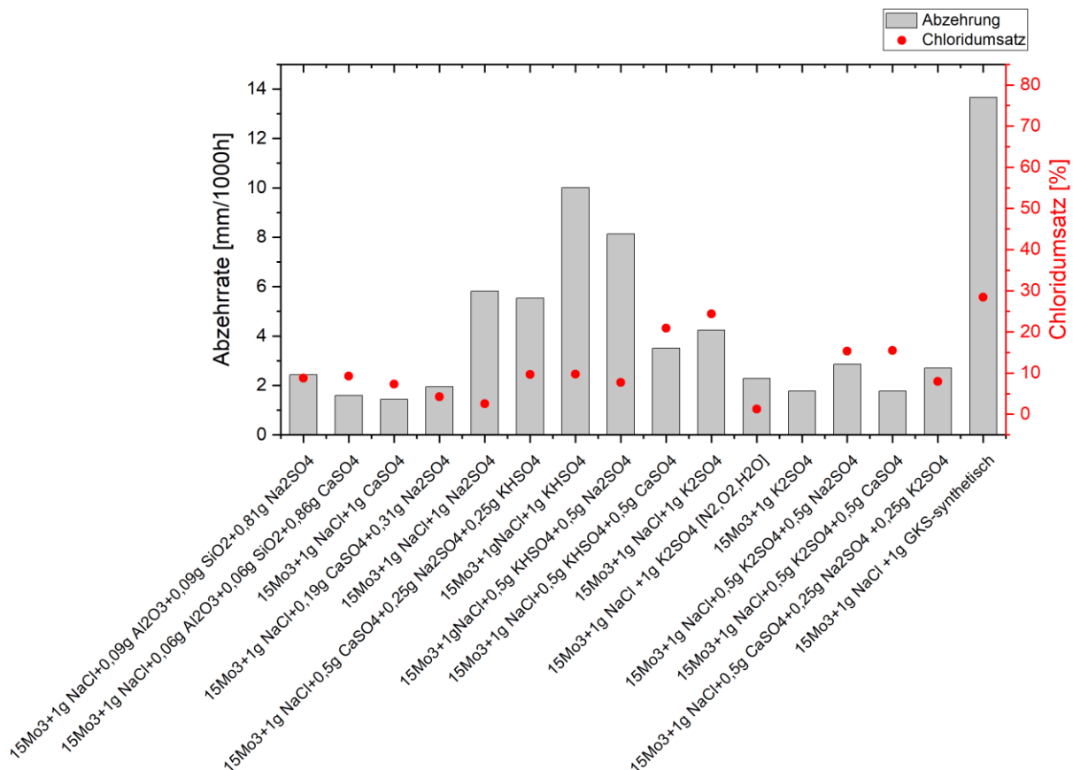
Abbildung 36: Laborexperimente: Stahl+NaCl mit Zusätzen unterschiedlicher Sulfat-(Oxid)-Gemische, Umsatz in [%] (rot) und Korrosion [mm/1000h] (grau) bei 600°C, 4 Stunden, [N 2 , O 2 , H 2 O, SO 2 ]
