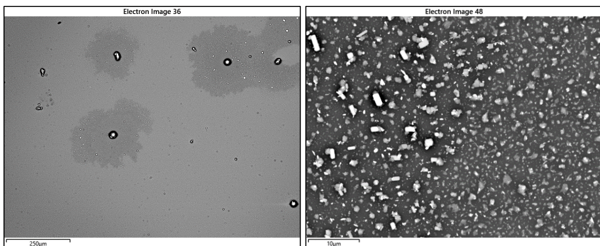
Abbildung 120: Partikelprobenahme MVV Gersthofen; REM-Aufnahmen, Versuchstag mit Additiv, Position nach Endüberhitzer, Sondentemperatur 380°C, Anströmseite, 10s im Rauchgas, niedrige und hohe Vergrößerung
