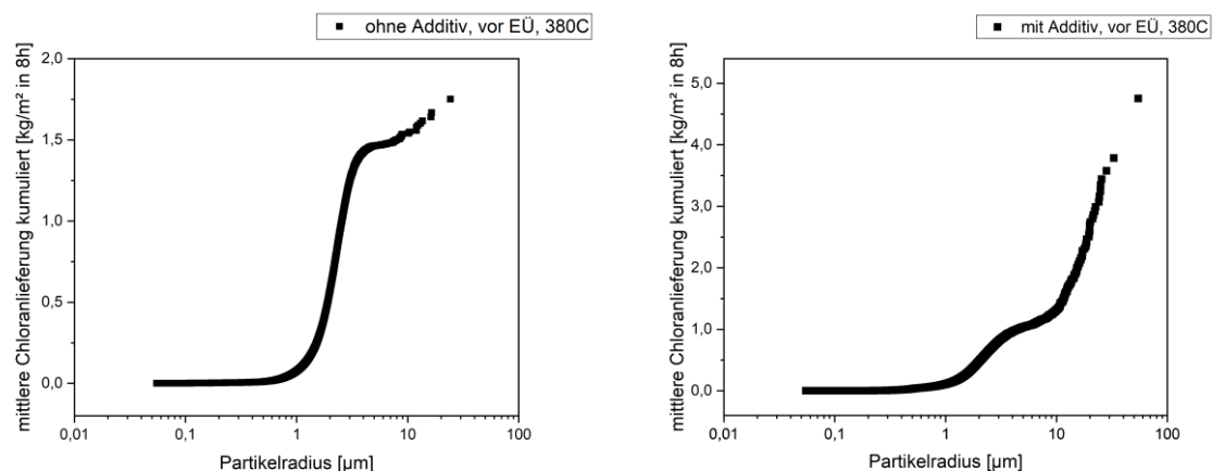
Abbildung 138: mittlere Chloranlieferung kumuliert, nach 8h, ohne und mit Additivdosierung, MVV Gersthofer, vor Endüberhitzer, Substrattemperatur 380°C, 10s im Rauchgas
