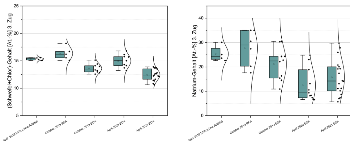
Abbildung 87: EDX-Belagsanalysen 3. Zug, MVV Gersthofen, Revisionen April 2019 bis April 2021, Box-Plot der Elemente Summe Chlor+Schwefel (a) und Natrium (Ca-Gehalt herausgerechnet) (b)
