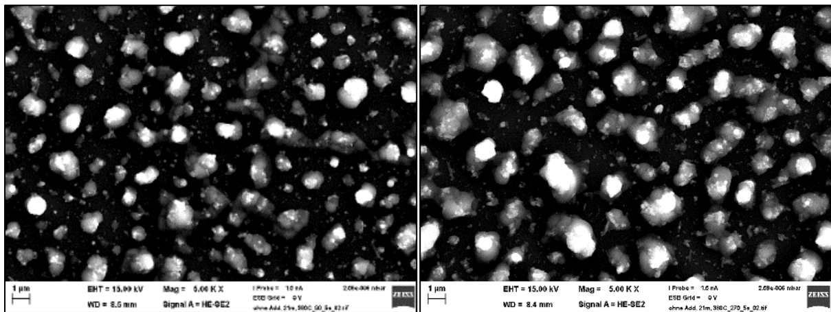
Abbildung 98: REM-Bild Partikelprobe ohne Additiv, nach EÜ, 380°C, 5s Flanke 90° (a) und Flanke 270° (b)
