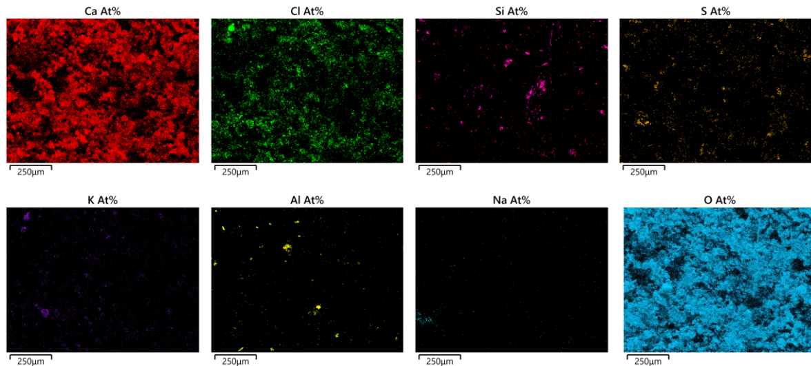
Abbildung 126: EDX-Mapping MHKW Rosenheim, mit Additiv, nach EÜ, Substrattemperatur 380°C, Anströmseite, 15min im Rauchgas
