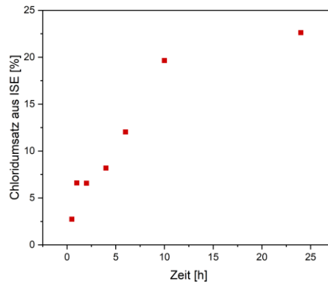
Abbildung 46: Zeitreihe Absorptionskinetik NaCl+Kaolin, Atmosphäre [N 2 , O 2 , H 2 O], 600°C, Umsatz bestimmt aus HCl-Freisetzung mittels ISE
