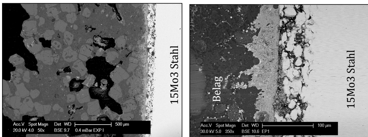
Abbildung 38: REM-Aufnahmen der Probe 15Mo3+1gNaCl+1gGKS-Belag bei 600°C, 4h und voller Atmosphäre, Übersichtsaufnahme des Belags (a) und Detailansicht der Korrosionsfront (b)
