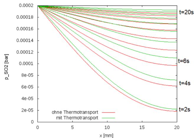
Abbildung 6: Berechnungen zur Gasdiffusion innerhalb des Belags entlang eines Temperaturgradienten von 873K bis 673K, ohne und mit Thermotransport, Porosität 10%, ( SO_2=200 ppm, O_2=8 %, N_2=80 %, Cl_2=1500 ppm, HCl=1500 ppm, H_2O=10 %) (Haider et al. 2017)
