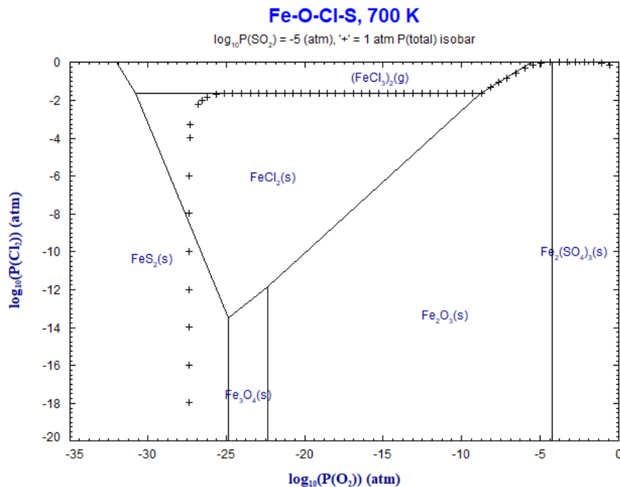
Abbildung 150: Stabilitätsdiagramm für Fe-O-Cl-S mit konstantem \text{SO}_2 = 10^{-5} \text{ atm} bei rund 430^\circ\text{C} (Bale et al. 2016)
