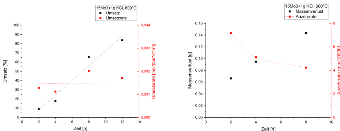
Abbildung 26: Zeitreihen für (a) den Umsatz des Salzes (in Prozent und als Umsatzrate [\text{mol}/(\text{bar}\cdot\text{s}\cdot\text{m}^2)] ) und (b) die Abzehrung des Stahls (Massenverlust in Gramm und Abzehrrate in [\text{mm}/1000\text{h}] ) für 15Mo3 mit 1g KCl unter [\text{N}_2, \text{O}_2, \text{H}_2\text{O} und \text{SO}_2]
