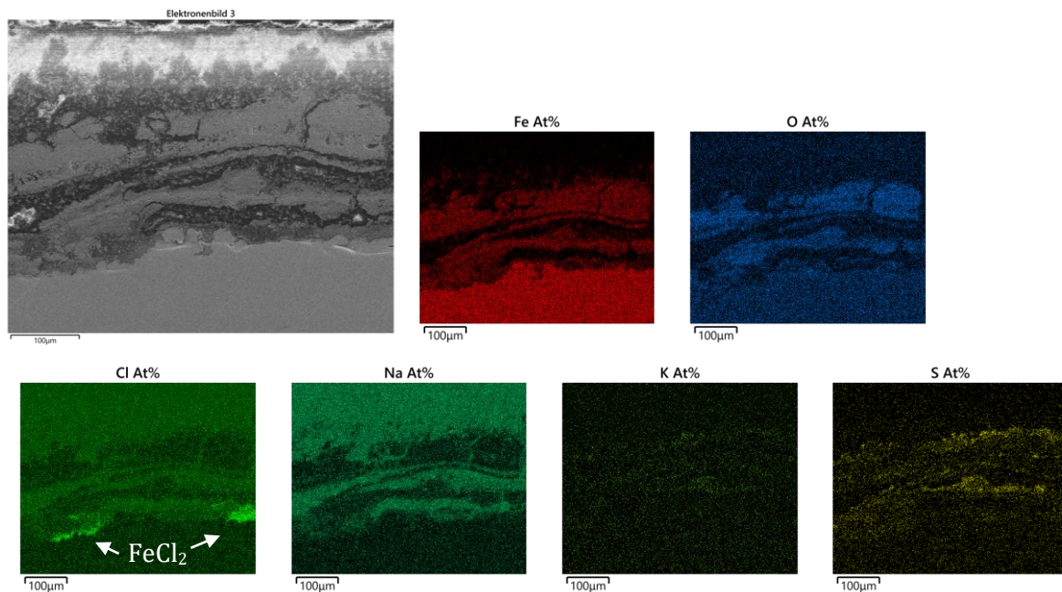
Abbildung 93: REM/EDX-Aufnahme der Korrosionsfront Austritt Überhitzer 2, MVV Gersthofen, (Kontrastgrenzen Fe und O: 50 At.-%, Cl, Na, K und S: 15 At.-%)
