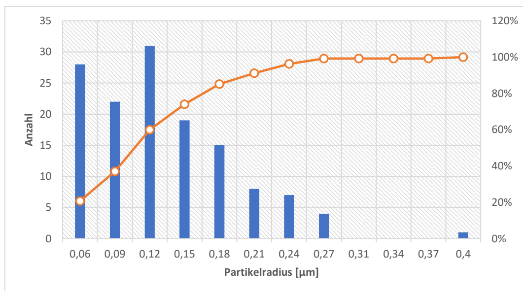
Abbildung 105: Partikelradius gegen Anzahl der Probe ohne Additiv, oberhalb EÜ, 380°C, 10s Abströmseite
