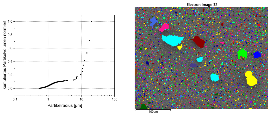
Abbildung 134: (a) kumuliertes Partikelvolumen (normiert) für einen Anteil der Partikel, MVV Gersthofen, mit Additiv, vor EÜ, Substrattemperatur 380°C, 10s im Rauchgas, (b) Bildausschnitt für Partikelchemieauswertung, detektierte Partikelanzahl 3476
