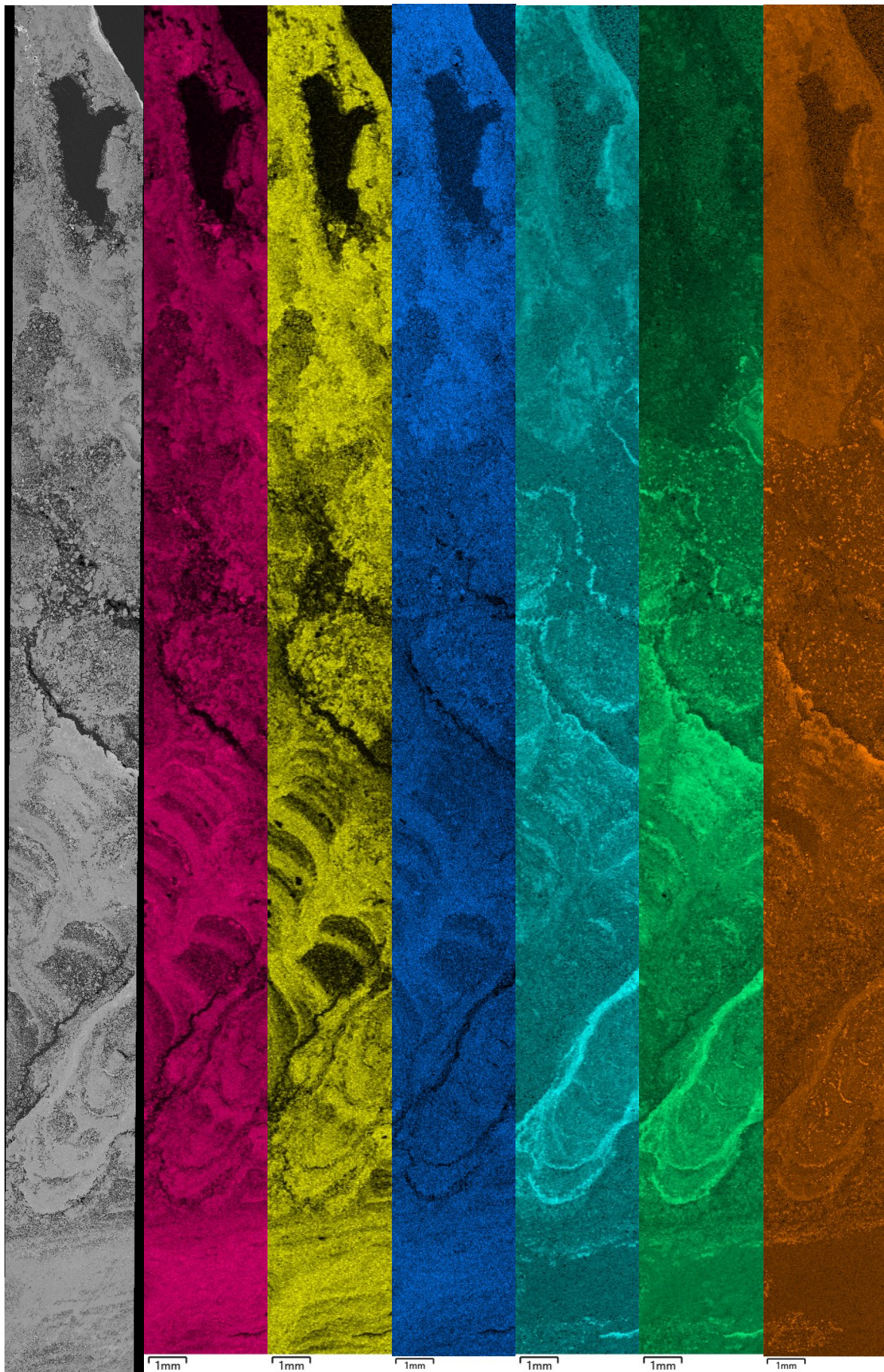
Abbildung 95: REM- und EDX-Scan durch einen Belagsbart von Überhitzer 2, MVV Gersthofen, Revision Oktober 2019, Elemente Ca (pink), S (gelb), O (blau), Na (cyan), Cl (grün), K (orange)
