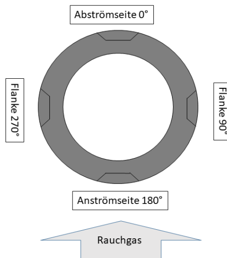
Abbildung 21: Skizze Sondenkopf mit Schwalbenschwanzfräsungen, Waferpositionen am Rohr, im Falle der Anlage MVV Gersthofen mit Rauchgas von unten
