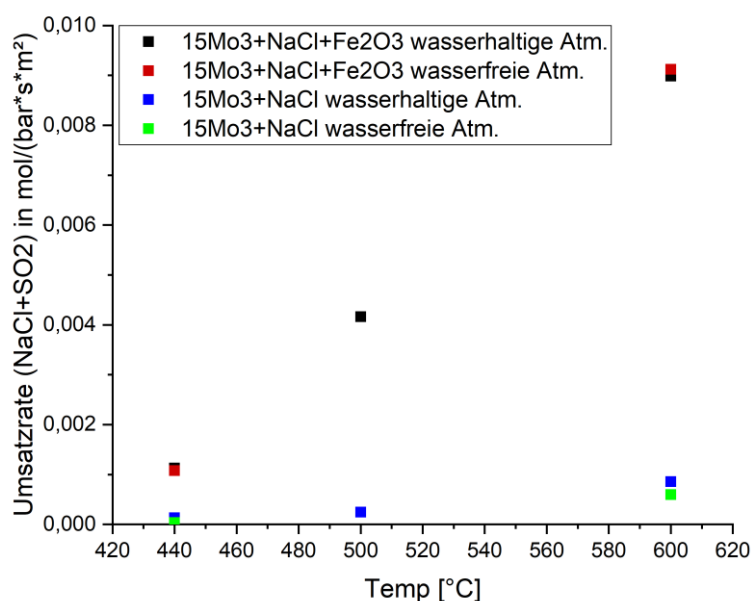
Abbildung 29: Sulfatierungsrate der Experimente von Stahl mit NaCl ohne und mit Eisenoxidzusatz, in wasserhaltiger und wasserfreier Atmosphäre, in Abhängigkeit von der Temperatur
