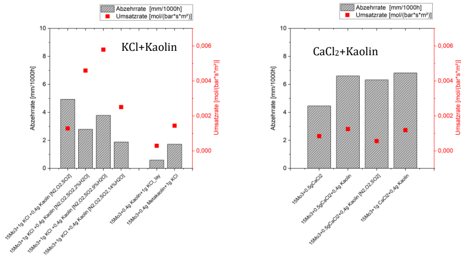
Abbildung 50: Laborexperimente mit Stahl+KCl und Zugabe von Kaolin bei 600°C für 4h
