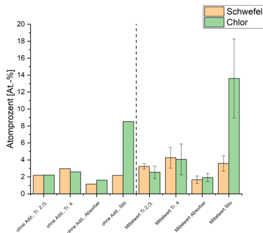
Abbildung 141: Chlor- und Schwefelgehalte in den Aschen: Trichter 2./3. Zug, 4. Zug, Absorber und Silo, ohne Additiv Januar 22 und mit Additiv Mittelwert aus Januar 22, Oktober 21
