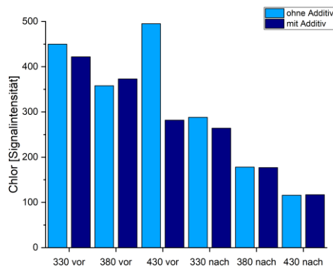
Abbildung 131: EDX Signalintensitäten für Chlor und Schwefel, vor und nach EÜ, ohne und mit Additiv für die unterschiedlichen Substrattemperaturen 330°C, 380°C, 430°C
