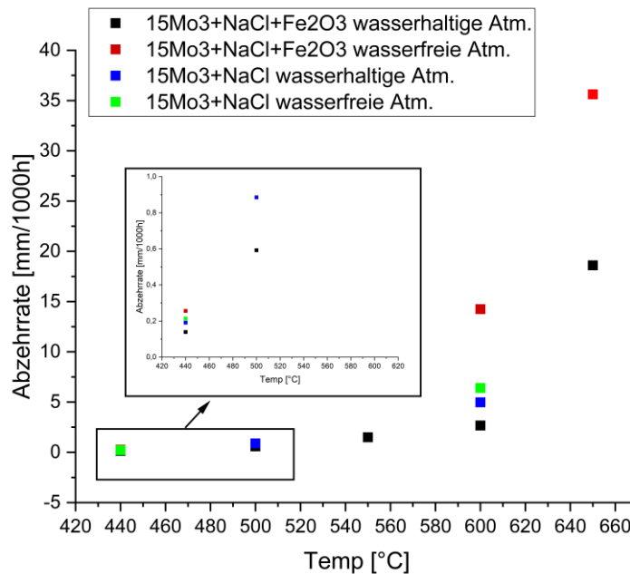
Abbildung 30: Metallabzehrung der Experimente von Stahl mit NaCl ohne und mit Eisenoxidzusatz, in wasserhaltiger und wasserfreier Atmosphäre, in Abhängigkeit von der Temperatur (rechts: Detailansicht der niedrigen Temperaturen)
