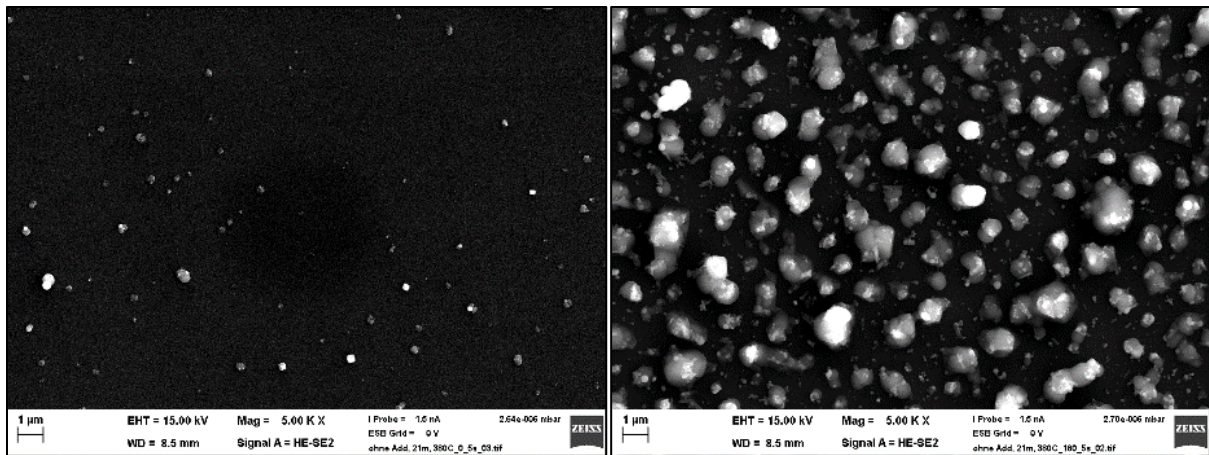
Abbildung 97: REM-Bild Partikelprobe ohne Additiv, nach EÜ, 380°C, 5s Abströmseite (a) und Anströmseite (b)
