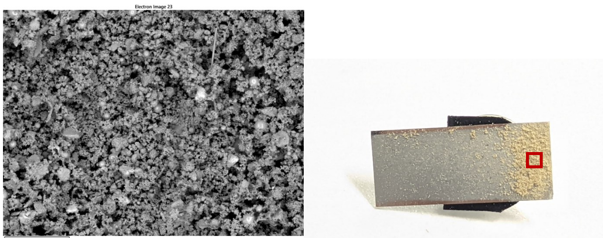
Abbildung 125: (a) REM-Aufnahmen Partikelproben, MHKW Rosenheim, mit Additiv, nach EÜ, Substrattemperatur 380°C, Anströmseite, 15min im Rauchgas, (b) Messposition auf Wafer mit Partikeldeposition 15 min im Rauchgas (nur der rechte Bereich)
