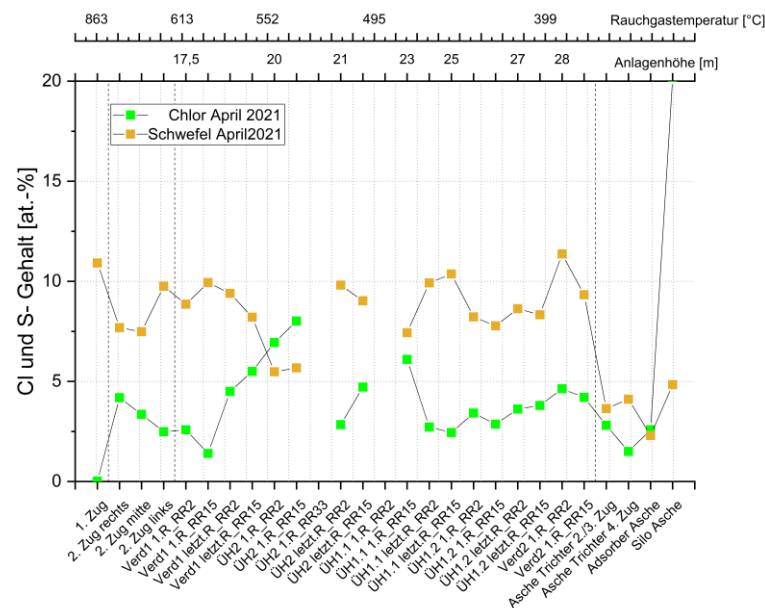
Abbildung 84: EDX-Belags- und Ascheanalysen Kraftwerk MVV Gersthofen, Probenahme April 2021, Chlor und Schwefel entlang der Anlage
