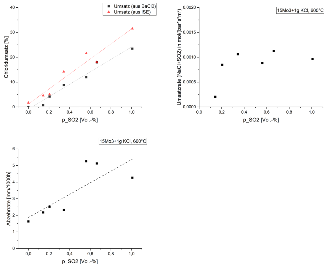
Abbildung 28: Variation des SO 2 -Partialdrucks für den Umsatz des Salzes in Prozent (a), die Umsatzrate von 15Mo3 mit 1g KCl unter voller Atmosphäre (b) und die Abzehrung des Stahls (c)
