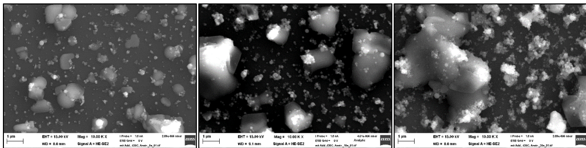
Abbildung 110: REM-Bilder Partikelprobe mit Additiv, nach EÜ, 430°C, Anströmseite, Zeitreihe von 5s, 10s und 20s im Rauchgasstrom
