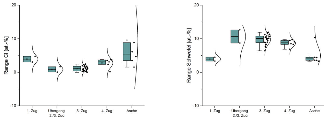
Abbildung 76: EDX-Belags- und Ascheanalysen GKS, Revision Oktober 2021, Box-Plot Chlor (ohne Gewebefilter: 32,6 At.-%) und Schwefel entlang der Anlage
