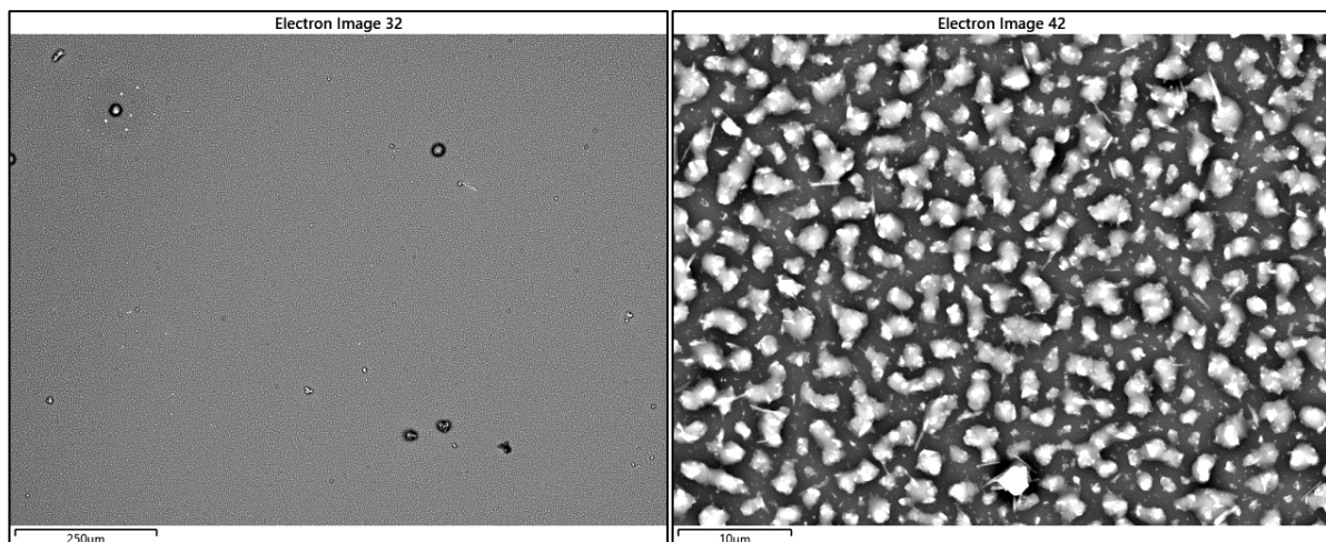
Abbildung 118: Partikelprobenahme MVV Gersthofen; REM-Aufnahmen, Versuchstag ohne Additiv, Position nach Endüberhitzer, Sondentemperatur 380°C, Anströmseite, 10s im Rauchgas, niedrige und hohe Vergrößerung
