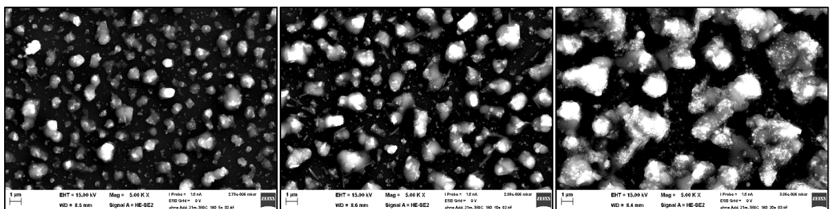
Abbildung 101: REM-Bilder Partikelprobe ohne Additiv, vor EÜ, 380°C, Anströmseite, Zeitreihe von 5s, 10s und 20s im Rauchgasstrom
