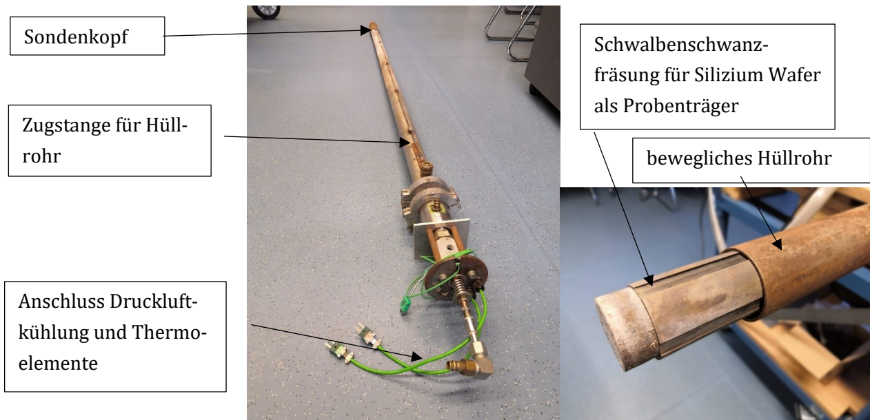
Abbildung 22: links: Druckluft-temperierte Messsonde zur Online-Partikelprobenahme; rechts: Sondenkopf mit Hüllrohr und unterschiedlichen Probenahmepositionen
