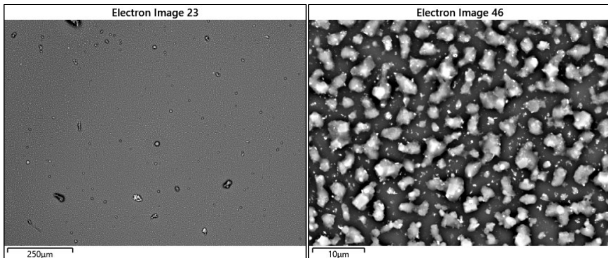
Abbildung 145: REM-Aufnahmen: Partikelproben MHKW Rosenheim, ohne Additiv, nach EÜ, Anströmseite, Substrattemperatur 380°C, 10s im Rauchgas
