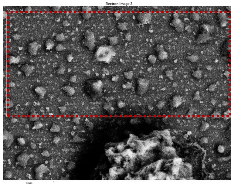
Abbildung 124: REM-Aufnahme (BSE-Detektor) der Probe mit Additiv, oberhalb EÜ, 430°C, Anströmseite, 10s, t.-%2.500-fache Vergrößerung mit eingezeichnetem Teilspektrum (Spektrum 13)
