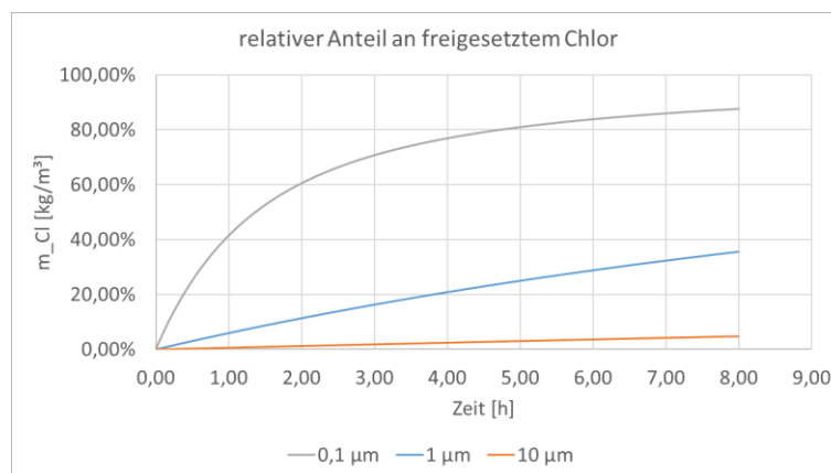
Abbildung 148: relativer Anteil an freigesetztem Chlor aus den unterschiedlichen Partikelgrößen, berechnet aus dem Verhältnis der mittleren freigesetzten Masse Chlor zur mittleren Chloranlieferung zur Zeit t
