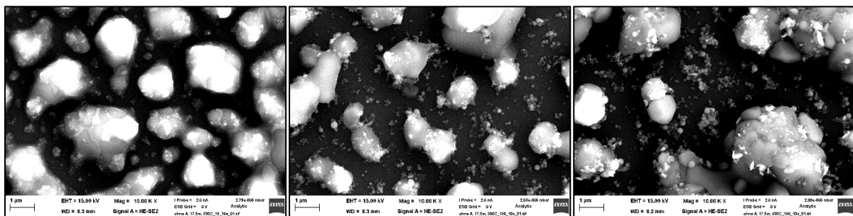
Abbildung 107: REM-Bilder Partikelprobe ohne Additiv, vor EÜ, 10s, Anströmseite, Temperaturreihe von 330°C, 380°C und 430°C als Substrattemperatur
