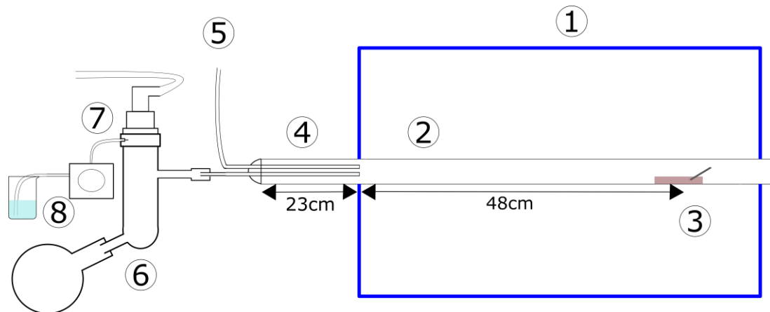
Abbildung 12: schematische Darstellung des Versuchsaufbaus zur Erzeugung und Abscheidung feiner Chloridpartikel; (1) Multizonenofen, (2) Quarzglasrohr, (3) Schlitten mit Siliziumwafer (2,0 x 1,0 cm), (4) Zwei-Wege Glaseinlass, (5) Trägergaseinlass, (6) Zerstäuber mit Kondensatauffang, (7) Schlauchpumpe, (8) Chlorldösung (50 ml: 1% NaCl) (Kroh 2021)
