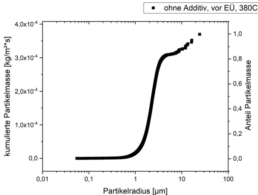
Abbildung 113: Partikelprobenahme MVV Gersthofen; kumulierte Partikelgrößenverteilung, ohne Additiv, Position vor Endüberhitzer, Substrattemperatur 380°C, Anströmseite, 10s im Rauchgas, ausgewertete Partikelzahl: 60.041
