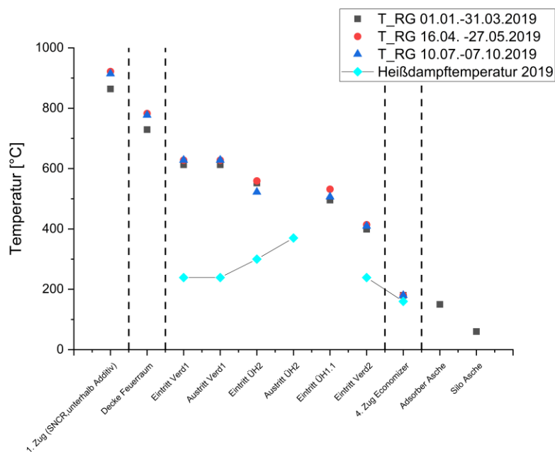
Abbildung 20: Temperaturverlauf Rohgas- und Heißdampftemperatur entlang der Anlage MVV Gersthofen, aus Anlagendaten
