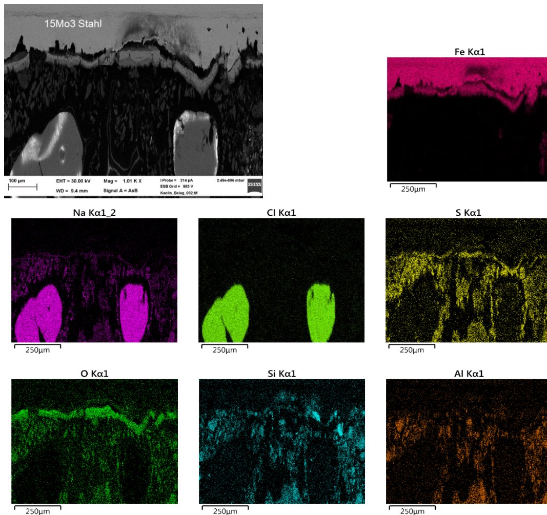
Abbildung 52: BSE- und EDX-Aufnahmen, Laborexperiment Stahl+NaCl+Kaolin, 600°C, 4h
