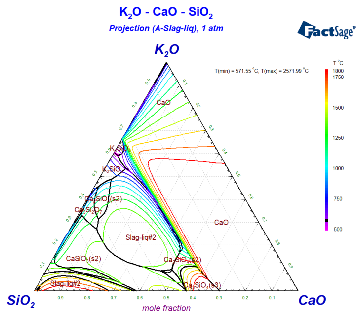
Abbildung 9: Liquidusprojektion \text{SiO}_2\text{-K}_2\text{O-CaO} (Bale et al. 2016)
