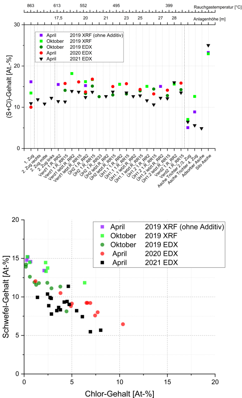
Abbildung 85: EDX-Belags- und Ascheanalysen Kraftwerk MVV Gersthofen, Revisionen April 2019 bis Oktober 2021, (a) Chlor+Schwefel entlang der Anlage; (b) Korrelation Schwefel zu Chlor im 3. Zug April 2019 (ohne Additiv) - April 2021 (mit Additiv)
