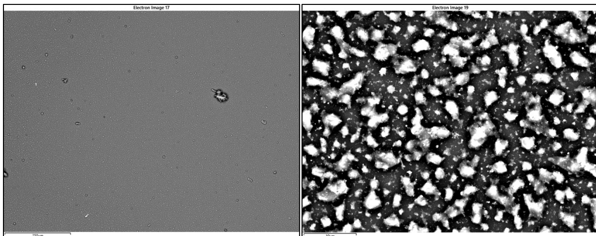
Abbildung 143: REM-Aufnahmen: Partikelproben MHKW Rosenheim, ohne Additiv, vor EÜ, Anströmseite, Substrattemperatur 380°C, 10s im Rauchgas
