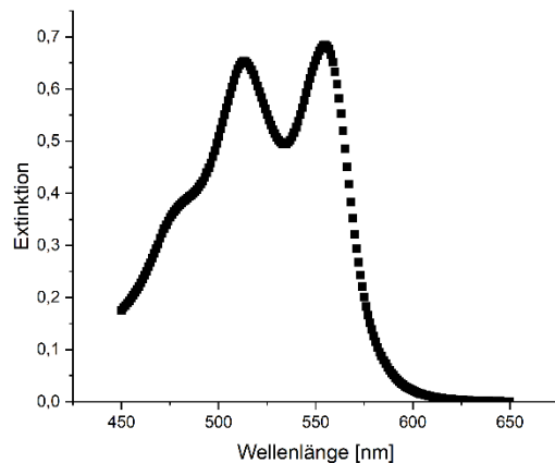
Abbildung 14: UV/Vis-Spektrum, Extinktion des DPD-Indikators nach Reaktion mit NaOCl-Lösung (0,0005%)
