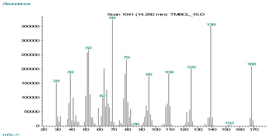
Abbildung 16: Massenspektrum von TMB
