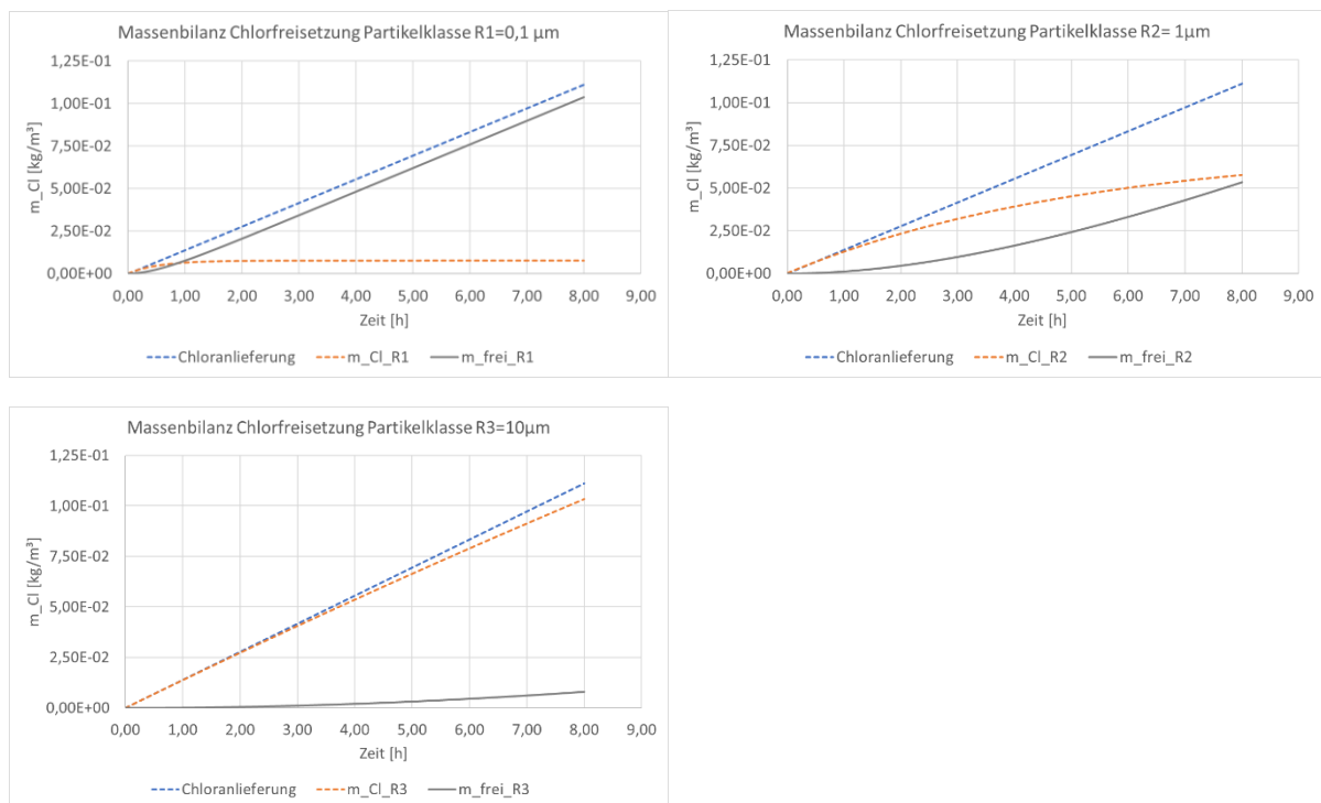
Abbildung 147: Chloranlieferung (blau), verbleibende Chlormasse m_{Cl}(t) (orange) sowie freigesetzte Chlormasse m_{frei} (grau) für Partikel der Größenklasse 0,1\ \mu\text{m} , 1\ \mu\text{m} und 10\ \mu\text{m}
