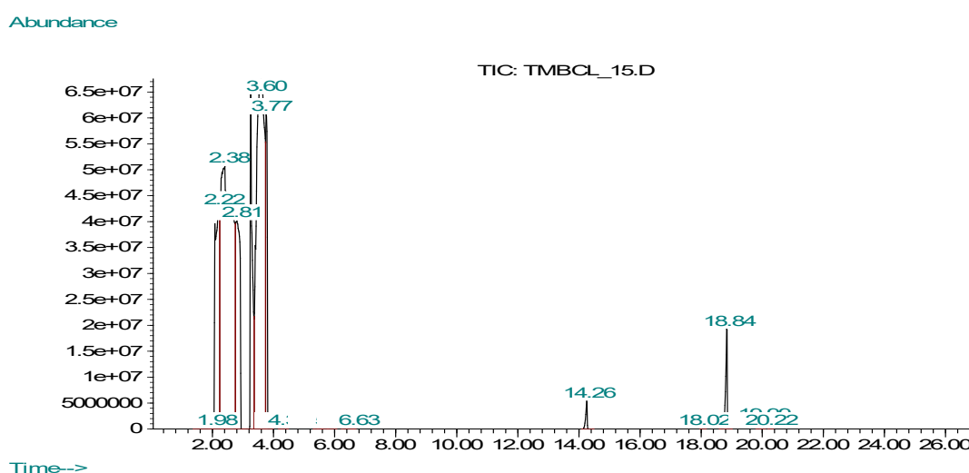
Abbildung 15: Chromatogramm von TMB in Ethylacetat, beaufschlagt mit \text{Cl}_2
