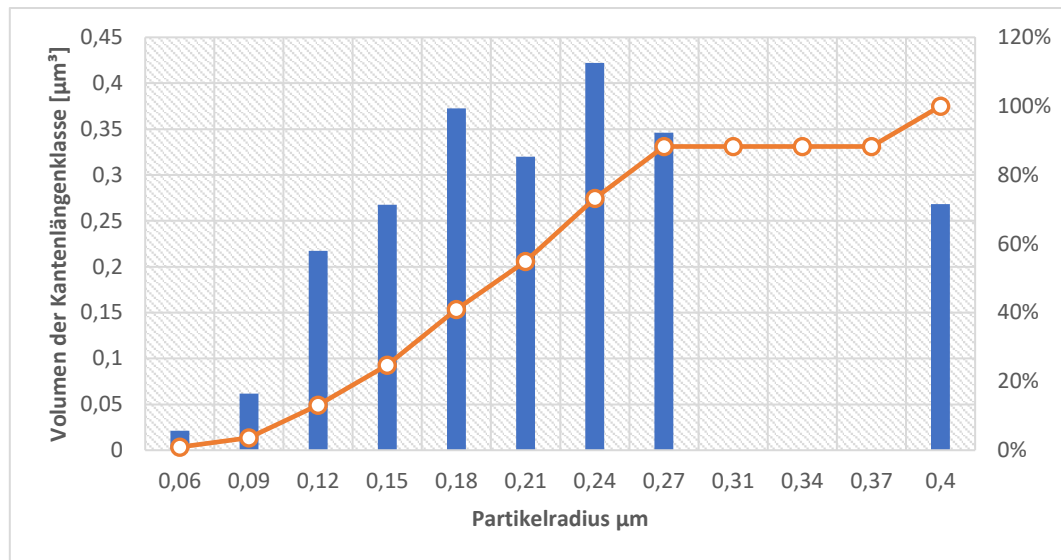
Abbildung 106: Partikelradius gegen Volumen der Kantenlängenklasse für die Probe ohne Additiv, oberhalb EÜ, 380°C, 10s Abströmseite
