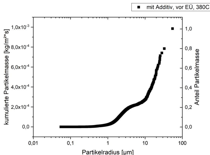
Abbildung 115: Partikelprobenahme MVV Gersthofen; kumulierte Partikelgrößenverteilung, Versuchstag mit Additiv, Position vor Endüberhitzer, Sondentemperatur 380^\circ\text{C} , Anströmseite, 10s im Rauchgas, ausgewertete Partikelzahl: 53.557
