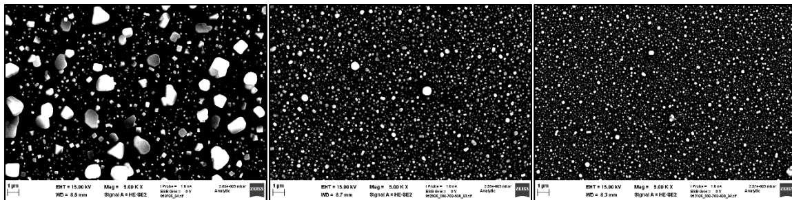
Abbildung 66: REM-Aufnahmen der abgeschiedenen NaCl-Partikel im Gastemperaturgradienten von 800-700 °C auf Siliziumplättchen mit Substrattemperatur von a) 600°C, b) 500°C und c) 400°C
