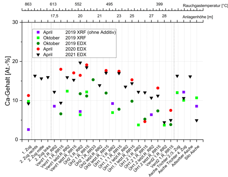
Abbildung 82: EDX Belags- und Ascheanalysen Kraftwerk MVV Gersthofen, Revisionen April 2019 bis Oktober 2021, Calcium entlang der Anlage
