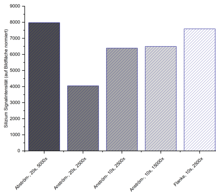
Abbildung 127: EDX-Signalintensität des Siliziumsubstrats der Probe ohne Additiv, nach EÜ, 430°C für Abströmseite (0°), Anströmseite (180°) und Flanke (90°), bei unterschiedlich langen Zeiten und für verschiedene Vergrößerungen der REM-Aufnahmen
