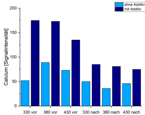
Abbildung 130: EDX-Signalintensitäten für Calcium, vor und nach EÜ, ohne und mit Additiv für die unterschiedlichen Substrattemperaturen 330°C, 380°C, 430°C
