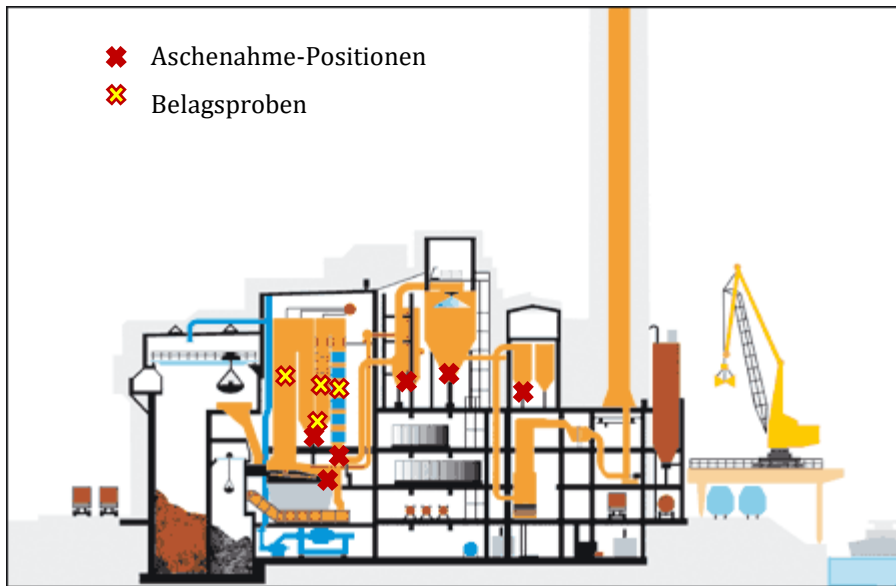
Abbildung 18: Schnitt durch das Gemeinschaftskraftwerk Schweinfurt, Aschenahme und Belagsproben-Positionen (im 3. und 4. Zug an weiteren Positionen) (GKS Schweinfurt 2022)
