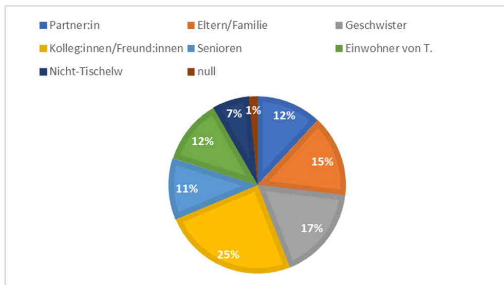
Figure 16: Kontexte FRIAUL
