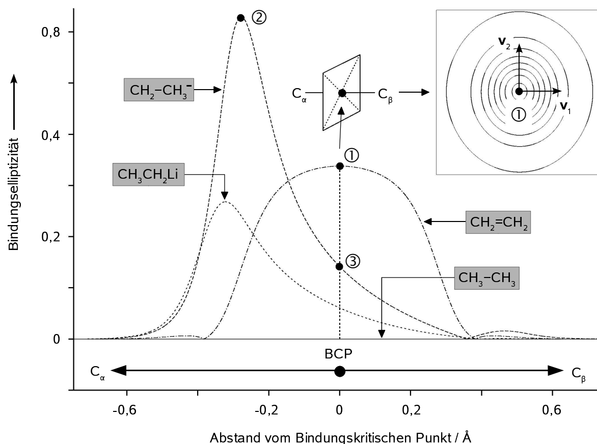
Abbildung 4.7: Theoretische Elliptizitätsprofile entlang des C_\alpha - C_\beta -Bindungspfades in [\text{CH}_2\text{CH}_3]^- ( 30 ) und \text{LiCH}_2\text{CH}_3 ( 33 ) im Vergleich zu \text{C}_2\text{H}_6 ( 29 ) sowie \text{C}_2\text{H}_4 ( 31 ). Die Definition von \varepsilon ist in der rechten oberen Ecke durch die Konturliniendarstellung von \rho(\mathbf{r}) in der Ebene gezeigt, die senkrecht zum BP durch den BCP der C-C-Bindung von 31 verläuft (Punkt ①). Demnach stellt \varepsilon ein Maß für die asphärische Ladungsdichteverteilung entlang des BP dar: \varepsilon = \lambda_1 / \lambda_2 - 1 ; \lambda_i bezeichnet dabei den Eigenwert des entsprechenden Eigenvektors \mathbf{v}_1 bzw. \mathbf{v}_2 der Hesse-Matrix von \rho(\mathbf{r}) (vgl. Abschnitt 3.3.2).
