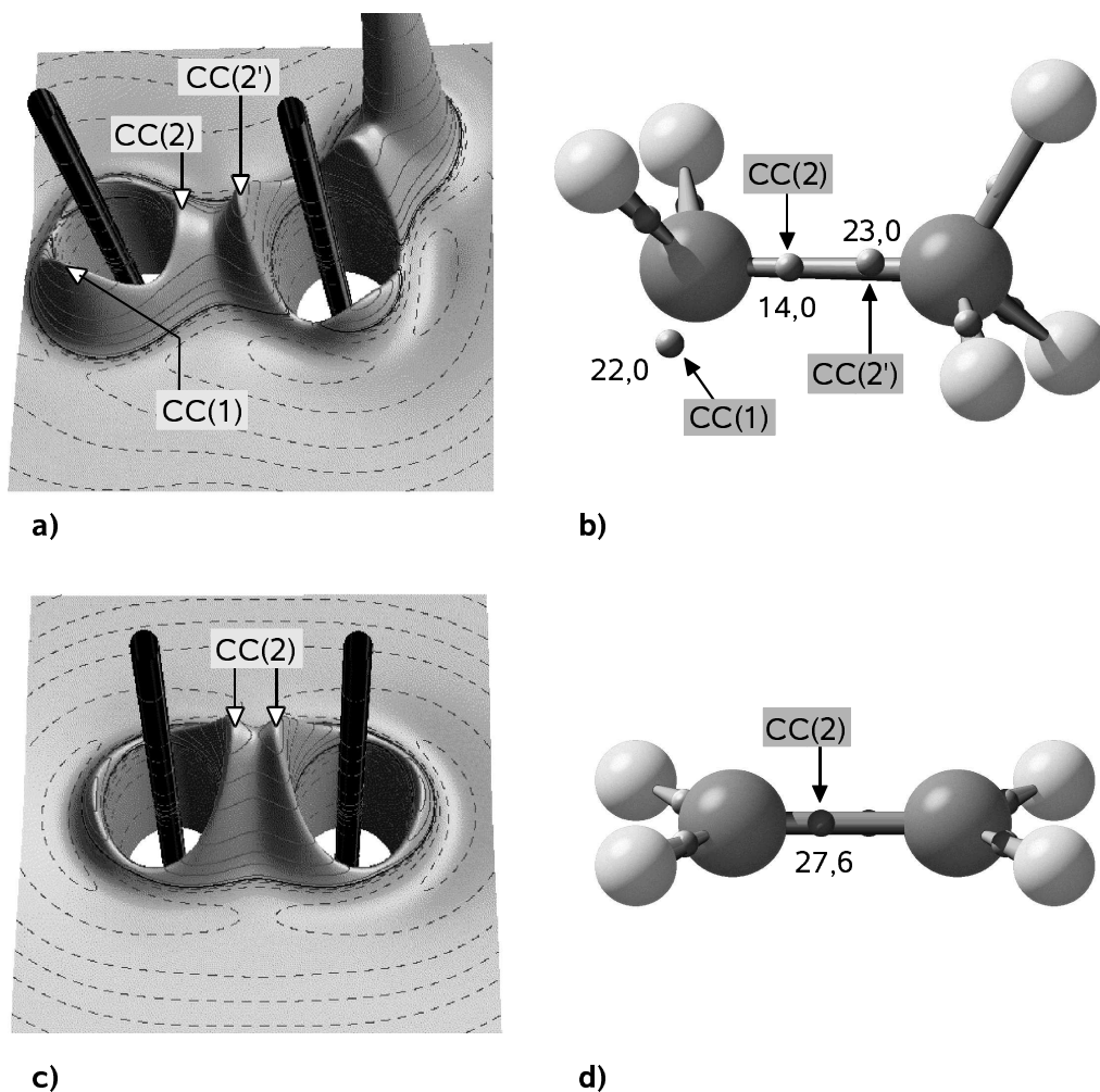
Abbildung 4.2: a), c) Reliefdarstellung der theoretischen Laplace-Funktion L(\mathbf{r}) in der C_\alpha-C_\beta-H -Ebene des Ethyl-Anions ( 30 ) bzw. der \sigma_v -Ebene des Ethens ( 31 ); für die Konturlinien gilt das in Abb. 4.1 gesagte; b), d) Moleküldarstellung von 30 bzw. 31 , aus der die räumliche Anordnung der CCs hervorgeht (Werte von L(\mathbf{r}) in \text{e}\text{\AA}^{-5} ).
