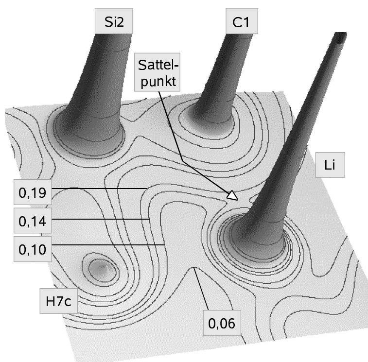
Abbildung 4.11: Reliefdarstellung der experimentellen totalen Ladungsdichte in der Li–C1–Si2-Ebene von 28 ; Konturlinien wurden für die Werte 0,06, 0,1, 0,14, 0,19, 0,4, 0,54, 0,8, 1,45, 1,85, 4, 8, und 20 eÅ –3 eingezeichnet. Die Position des Sattelpunktes bzw. BCPs zwischen Li und C1 ist durch einen Pfeil markiert.
