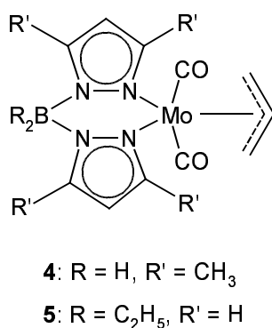
Abbildung 2.2: Strukturvorschlag Trofimenkos für die Pyrazolylboratkomplexe 4 und 5 , für die er Nicht-Edelgas-Konfigurationen postulierte.
