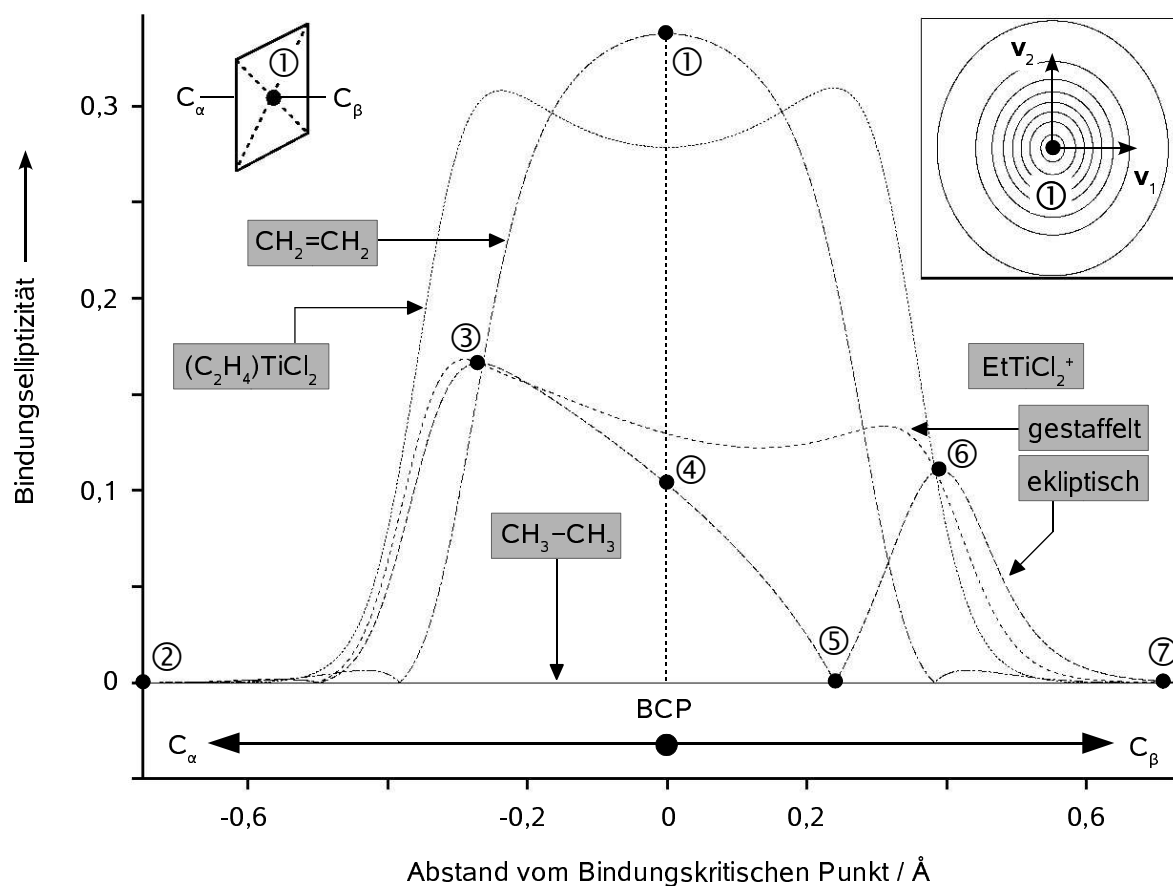
Abbildung 5.6: Berechnete Elliptizitätsprofile entlang des C_\alpha-C_\beta -Bindungspfad in [EtTiCl_2]^+ ( 42a : ekliptische, 42b : gestaffelte Konformation) im Vergleich zu C_2H_6 ( 29 ), C_2H_4 ( 31 ) und (\eta^2-C_2H_4)TiCl_2 ( 43 ). In der rechten oberen Ecke ist die Ladungsdichte in der Ebene gezeigt, die orthogonal zum BP durch den BCP von 31 verläuft; v_1 und v_2 stellen die Eigenvektoren der Hesse-Matrix von \rho(r) dar; für eine Definition der Elliptizität \epsilon siehe Abschnitt 3.3.2.
