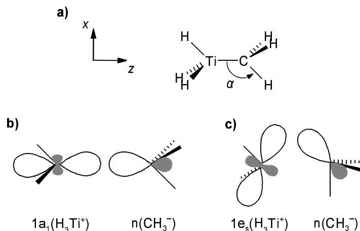
Abbildung 2.14: Schematische Darstellung des tetraedrischen Modellsystems 24 (a) und der bei verschiedenen Geometrien beteiligten Fragmentorbitale von [\text{H}_3\text{Ti}]^+ und [\text{CH}_3]^- (b, c); Details dazu im Text.
