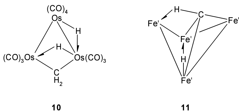
Abbildung 2.6: Schematische Darstellung der Neutronenstrukturmodelle des mehrkernigen Komplexes 10 sowie des Clusters 11 [ Fe' = Fe(CO)_3 ].
