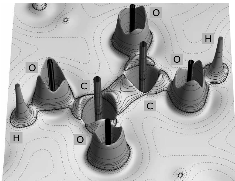
Abbildung 1.4: Reliefdarstellung des negativen Laplace-Operators der experimentellen Elektronendichte in der Molekülebene der Oxalsäure C 2 H 2 O 4 ; an den Orten chemischer Bindungen sowie freier Elektronenpaare sind Sattelpunkte bzw. Maxima von -\nabla^2\rho(\mathbf{r}) zu erkennen (für Details siehe Abschnitt 3).
