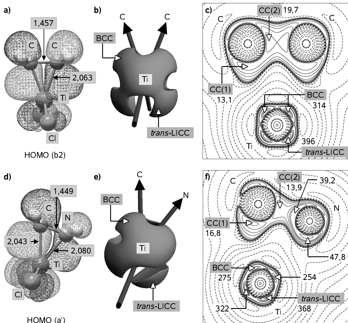
Abbildung 5.9: a), d) Darstellung der HOMOs von (\eta^2\text{-C}_2\text{H}_4)\text{TiCl}_2 ( 43 ) bzw. [(\eta^2\text{-CH}_2\text{NH}_2)\text{TiCl}_2]^+ ( 44 ); b), e) Darstellung der Iso-Oberflächen mit L(\mathbf{r}) = 160 \text{ e}\text{\AA}^{-5} für das Titanzentrum in 43 bzw. 44 ; c), f) Konturliniendarstellung des negativen Laplace-Operators der Ladungsdichte, L(\mathbf{r}) , in der Ebene Ti-C-X (X = C, N) von 43 bzw. 44 ; für die Konturlinien gilt (mit Ausnahme einer Extralinie bei 200 \text{ e}\text{\AA}^{-5} ) das in Abb. 5.1 gesagte.
