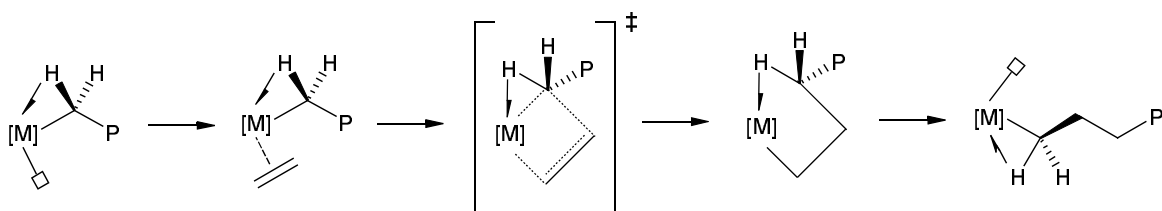
(3) Modifizierter Green-Rooney-Mechanismus [1, 8]
