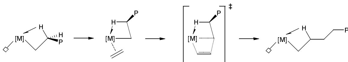
(4) Mechanismus nach T. Ziegler bei Rückseiten-Angriff [9]
