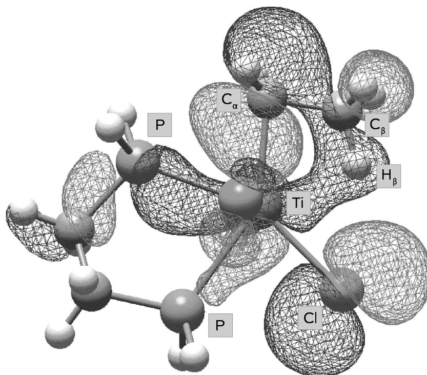
Abbildung 2.15: Darstellung des HOMO von EtTiCl_3(dmpe) ( 7 ). [58, 44]
