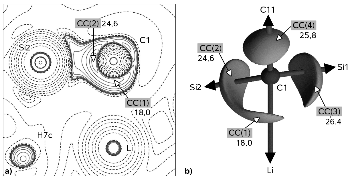
Abbildung 4.12: a) Konturliniendarstellung des experimentellen, negativen Laplace-Operators in der Li-C1-Si2-Ebene von 28 ; für die Werte der Konturlinien gilt dabei das in Abb. 4.1 gesagte; durchgezogene/gestrichelte Linien entsprechen positiven/negativen Werten von L(\mathbf{r}) ; b) Dreidimensionale Darstellung der Bereiche mit L(\mathbf{r}) = 17 \text{ e}\text{\AA}^{-5} um C1, durch die das beinahe Verschmelzen der beiden Ladungskonzentrationen CC(1) und CC(2) und damit die Elektronendelokalisierung deutlich wird.
