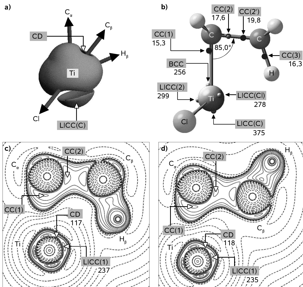
Abbildung 5.7: a) Darstellung der Iso-Oberfläche mit L(r) = 150 \text{ eÅ}^{-5} für das Titanzentrum in 42a ; b) DFT-Modell von 42a , aus der die relative Anordnung der CCs hervorgeht; c), d) Konturlinien-darstellung von L(r) in der Molekülebene Ti-C_\alpha-C_\beta-H_\beta von 42a bzw. 42b ; für die Konturlinien gilt (mit Ausnahme einer Extralinie bei 200 \text{ eÅ}^{-5} ) das in Abb. 5.1 gesagte.
