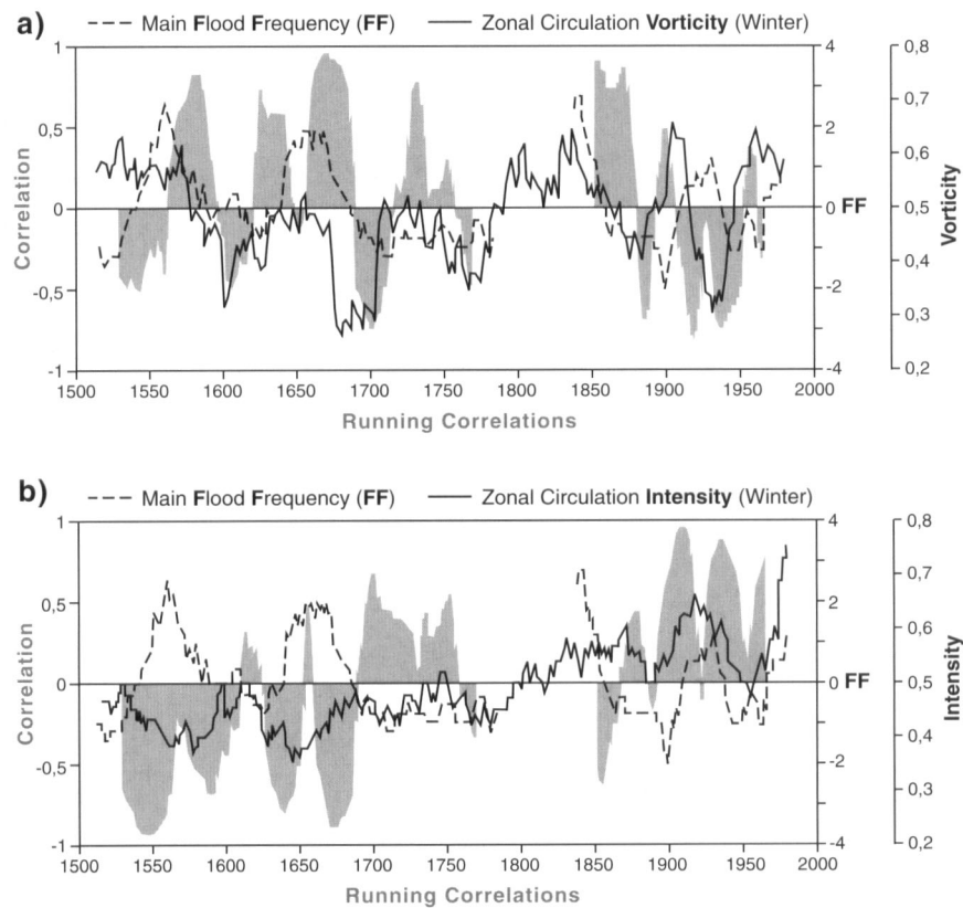
Fig. 9: 31-year running mean of the flood frequencies during winter at the river Main (dashed lines) and of two important circulation indices, determined in the central European area for the large-scale zonal, NAO-like circulation on Fig. 8a (JACOBET et al. 2002): Relative vorticity (full line on Fig. 9a) and pressure gradient intensity between the mode dependent-centres of action (full line on Fig. 9b). Shaded areas represent the running correlations between the two represented curves 31-jährige gleitende Mittel der winterlichen Fluthäufigkeiten im Gebiet des Mains (gestrichelte Linien) und von zwei wichtigen Zirkulationsindizes, welche für den Raum Mitteleuropa für die Zonalzirkulation auf Fig. 8a gerechnet wurden (JACOBET et al. 2002): Relative Vorticity (geschlossene Linie in Fig. 9a) und Druckgradient zwischen den wichtigsten Aktionszentren (geschlossene Linie in Fig. 9b). Graue Flächen markieren je die gleitenden Korrelationen zwischen den beiden Kurven
