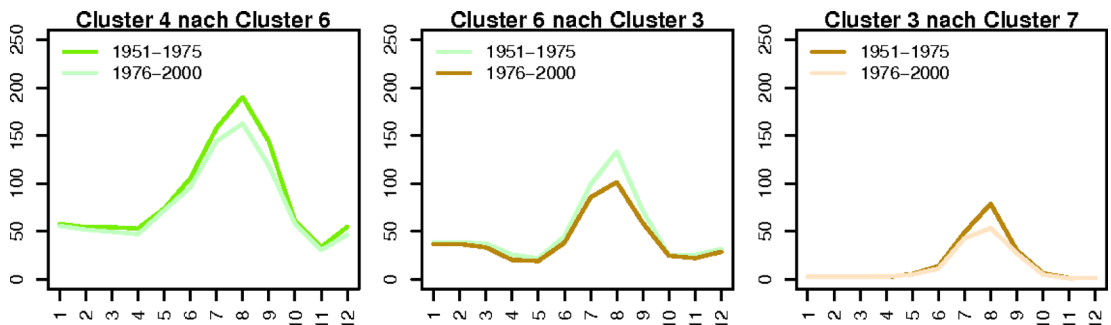
Abb. 3.1.9-4: Mittlere Niederschlagsjahresgänge derjenigen Rasterfelder, die in den Zeiträumen 1951–1975 und 1976–2000 verschiedenen Niederschlagsregimetypen zugeordnet wurden. Dargestellt für die 3 umfangreichsten Flächenumverteilungen aus Abb. 3.1.9-3 .
