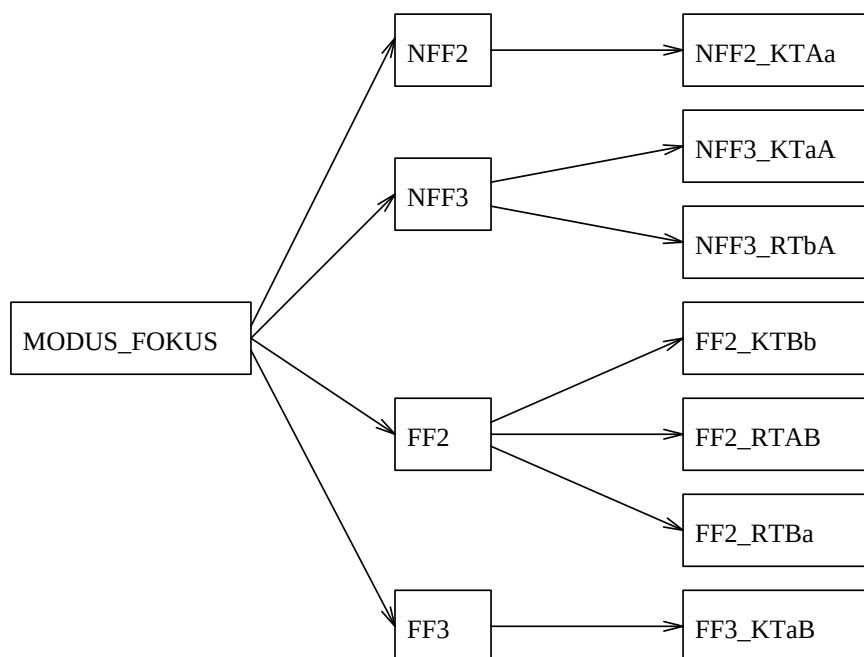
Abb. 9: Eingeschränktes Intonationsmodell
