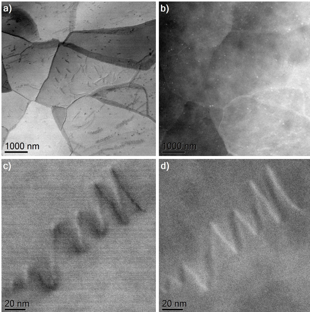
Abbildung 6.4: Helikale Versetzungslinien im T6-Zustand ( T_{\text{Hom}} = 530\text{ °C} , T_{\text{Aus}} = 165\text{ °C} , t_{\text{Aus}} = 2\text{ min} ); BF-STEM (links) und DF-STEM (rechts). Abb. a) und b): Übersicht der Kornstruktur. Abb. c) und d): Ansicht einer Versetzungshelix mit Blickrichtung senkrecht zur Helixachse.
