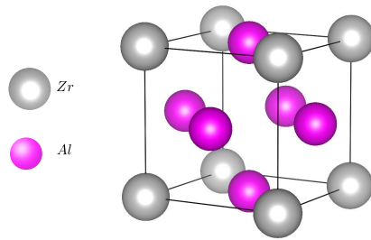
Abbildung 3.5: L1_2 -Struktur der \beta' -Phase ( Al_3Zr ).
