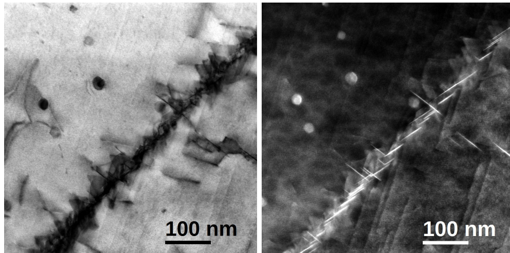
Abbildung 6.27: Probe: \epsilon = 0\% , T = 240\text{ °C} , t = 5\text{ Min.} STEM-Aufnahmen der Korngrenze zu Abbildung 6.26. Links Hellfeld-, rechts Dunkelfeld-Aufnahme. Deutlich zu erkennen sind die T_1 -Ausscheidungen, mit welchen die Korngrenze besetzt ist.
