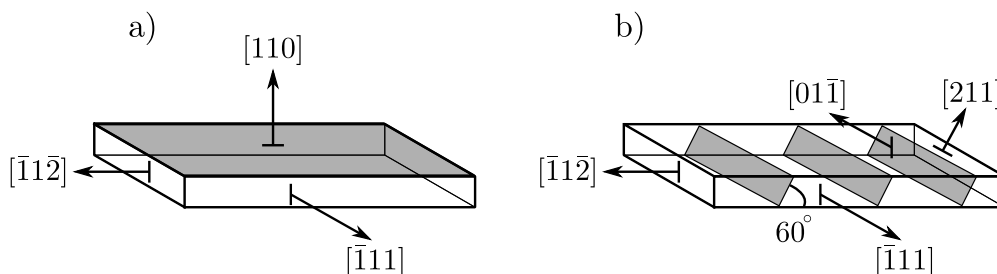
Abbildung 6.20: TEM-Probenpräparation in zwei unterschiedlichen Orientierungen: In a) [110]- und in b) [011]- Orientierung.
