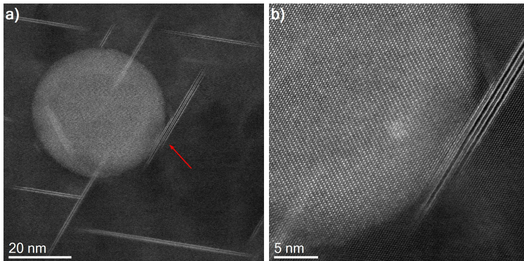
Abbildung 4.3: Hochaufgelöste DF-STEM-Aufnahme eines Al_3Zr -Dispersoids mit [110]_{Al} -Zonenachse. Abbildung (a): Sphärisches Al_3Zr -Dispersoid und von zwei Varianten der T_1 -Phase. Die an dem Dispersoid nukleierte T_1 -Platte (siehe Pfeil) ist dicker als die umliegenden T_1 -Ausscheidungen. Abbildung (b): Detailaufnahme Al_3Zr -Dispersoid mit nukleierter T_1 -Ausscheidung. [106]
