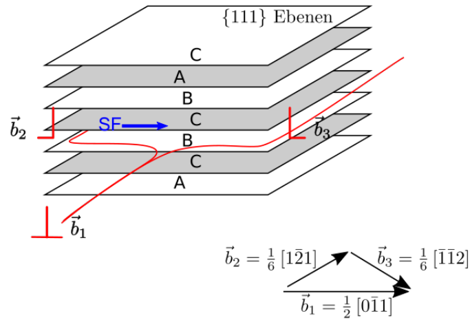
Abbildung 4.1: Entstehung eines intrinsischen Stapelfehlers durch Shockley-Partialversetzungen. Die Versetzung mit Burgersvektor \vec{b}_1 spaltet in zwei Partialversetzungen \vec{b}_2 und \vec{b}_3 vom Typ \frac{1}{6}\langle 112 \rangle auf. \vec{b}_2 erzeugt eine Verschiebung des darüber liegenden Gitters. Aus der Stapelabfolge A-B-C-A wird die Abfolge C-A-B-C-, darunter folgt das ungestörte Gitter -B-C-A. Durch die fehlende A-Ebene (siehe blauer Pfeil) entsteht ein Stapelfehler. Die Partialversetzung \vec{b}_3 stellt durch eine entgegengesetzte Verschiebung die ursprüngliche Abfolge wieder her. Zwischen den beiden Partialversetzungen hat sich ein Gitter mit hcp-Stapelabfolge B-C-B-C gebildet.
