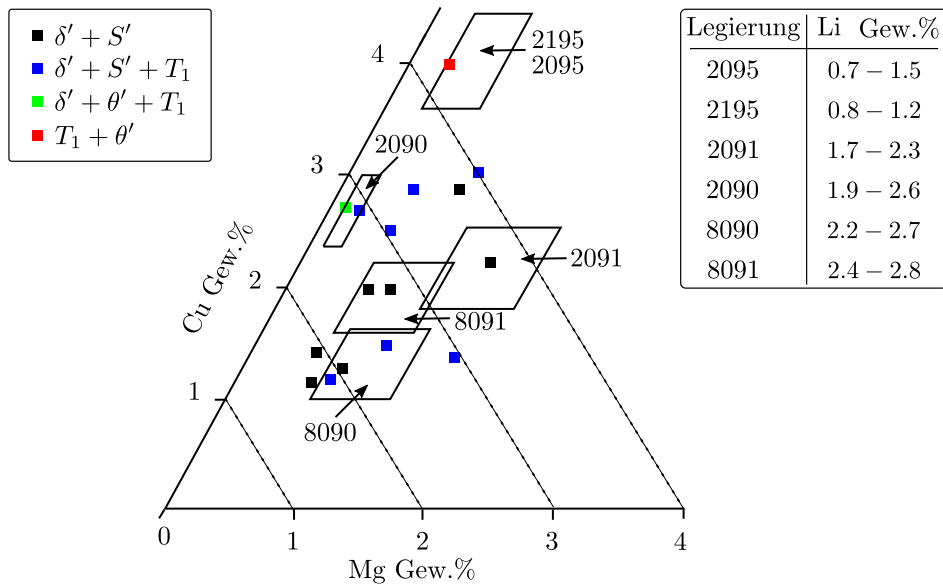
Abbildung 3.6: Ausscheidungsphasen in quaternären Al-Li-Cu-Mg-Legierungen nach einer Alterung bei 190°C. Nach [84, 85]. Die Legierung AA2195 weist die Phasen \text{Al}_2\text{CuLi} ( T_1 ) und \text{Al}_2\text{Cu} ( \theta' ) auf. In Legierungen mit einem Lithiumgehalt über 2 Gew.% bildet sich die lithiumhaltige Phase \delta' .
