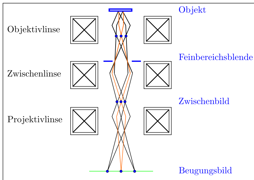
Abbildung 5.3: Strahlengang im Beugungsmodus. Das Beugungsbild aus der hinteren Brennebene der Objektive Linse wird abgebildet.
