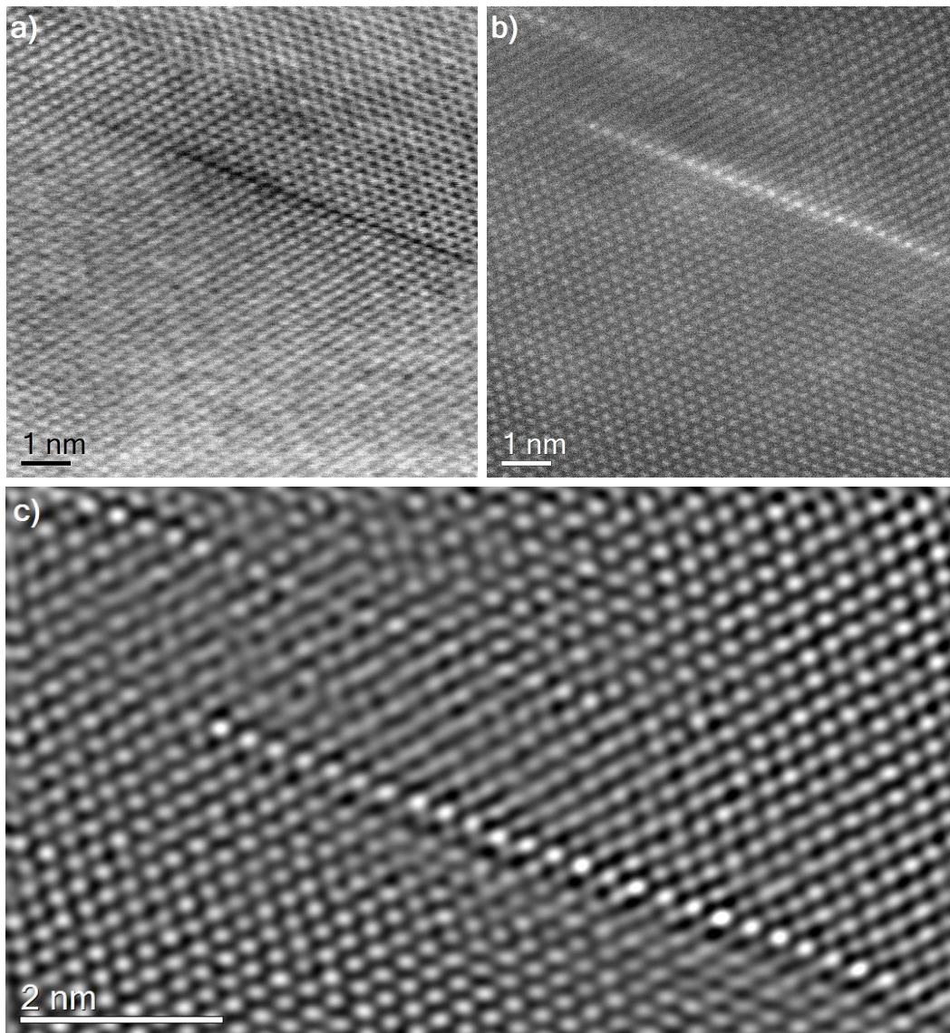
Abbildung 6.8: Hochaufgelöste STEM-Aufnahme einer GP-Zone mit [110]_{\text{Al}} -Zonenachse (Probe D, Tabelle 6.1). a) Im BF-STEM heben sich die schwereren Kupferatome der GP-Zone als dunkle Linie von der Aluminiummatrix ab; es können keine Versetzungen an der Ausscheidung und in deren Umgebung gefunden werden. b) Mittels HAADF-Detektor im DF-STEM lässt sich die GP-Zone atomar aufgelöst darstellen. Abbildung c) zeigt die fouriergefilterte DF-Aufnahme.
