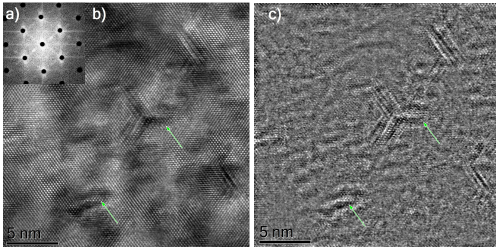
Abbildung 6.10: Mikrostruktur der Probe E ( T_{\text{Hom}}=510\text{ °C} , T_{\text{Aus}}=165\text{ °C} , t_{\text{Aus}}=30\text{ min} ). b) HRTEM mit a) FFT Inset, Zonenachse [110]_{\text{Al}} . c) Die IFFT Abbildung (ohne Aluminiumgitter) weist T_1 - und \theta' -Ausscheidungen (grüne Pfeile) auf.
