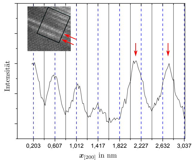
Abbildung 6.13: Ausschnitt aus 6.11, Probe B. Intensitätsprofil über zwei nukleierte Monolagen und das \text{Al}_3\text{Zr} -Dispersoid. Die Monolagen liegen phasenverschoben zur L_{12} -Struktur und haben einen Abstand von 0,64 nm; dies entspricht ca. dem dreifachen (200)-Netzebenenabstand in Aluminium ( d_{\{200\}} = 0,203 nm) bzw. zwei Netzebenen Aluminium zwischen den Monolagen. Bei dieser Anordnung handelt es sich damit nicht um eine GP(II)-Zone, bestehend aus zwei Monolagen Kupfer mit drei dazwischenliegenden (200)-Ebenen Aluminium.
