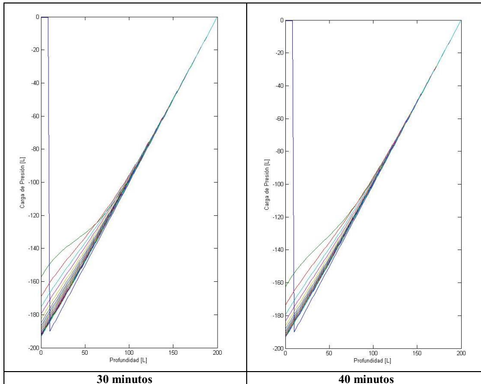
Fig. 4. Tendencia de la Carga de Presión a diferentes profundidades de suelo.
