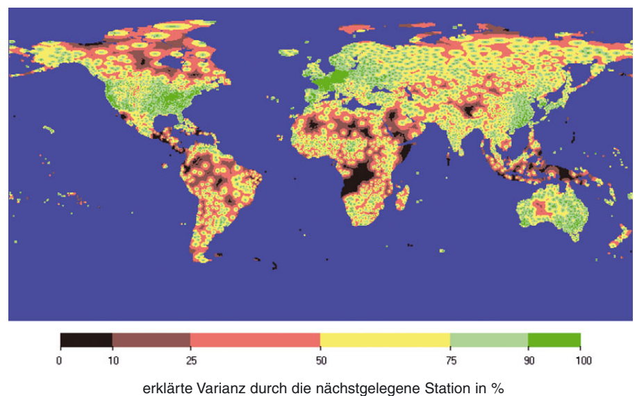
Abb. 4: Durch die nächstgelegene Station erklärter Varianzanteil der Januarniederschläge an jedem Gitterpunkt.
