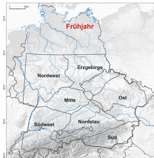
Abb. 4.4-1: Regionen ähnlicher Niederschlagsvariabilität, abgeleitet aus S-modalen Hauptkomponentenanalysen der täglichen Gitternetz-Niederschläge für Frühjahr und Sommer 1951-2006 (verändert nach HOMANN 2017).
