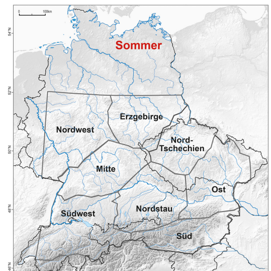
Abb. 4.4-1: Regionen ähnlicher Niederschlagsvariabilität, abgeleitet aus S-modalen Hauptkomponentenanalysen der täglichen Gitternetz-Niederschläge für Frühjahr und Sommer 1951-2006 (verändert nach HOMANN 2017).
