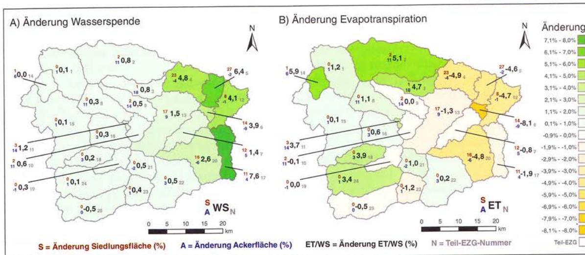
Abb. 2: Auswirkungen des vergangenen Landnutzungswandels auf Wasserspense (A) und Evapotranspiration (B) in den Teileinzugsgebieten des Untersuchungsgebiets
