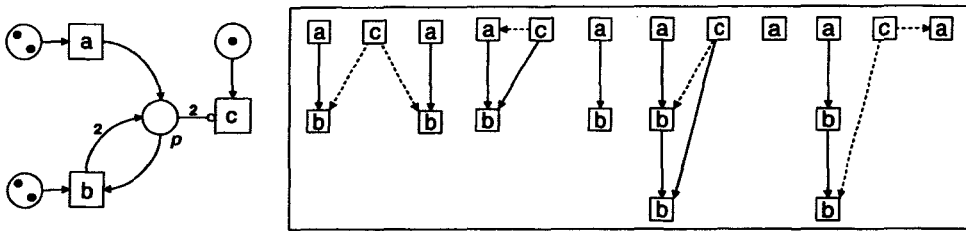
Abbildung 1: Ein STI-Netz mit seinen minimalen Ausführungen.
