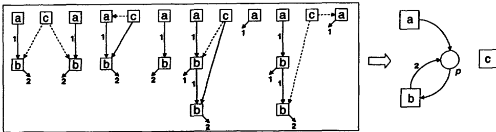
Abbildung 3: Eine mögliche Markenflussfunktion r bzgl. der BGOs aus Abbildung 1. Die Knoten v_0 bzw. v_m wurden weggelassen; die zugehörigen Kanten werden als Kanten ohne Anfangs- bzw. Endknoten dargestellt (und nur gezeichnet falls ihr Markenfluss ungleich null ist). Rechts ist die zugehörige Stelle noch ohne Inhibitor-kanten abgebildet.
