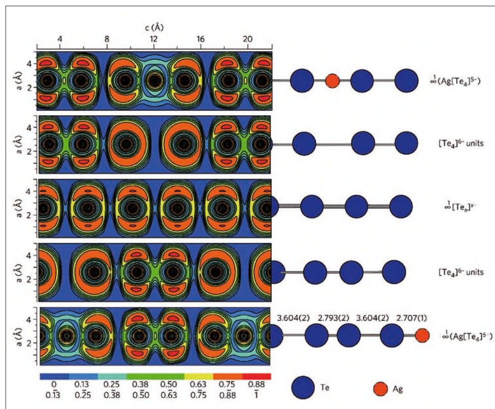
Abb. 1. ELF-Analyse der polyanionischen Teilstruktur von \text{Ag}_{10}\text{Te}_4\text{Br}_3 ; innerhalb der Struktur \text{Ag}_{10}\text{Te}_4\text{Br}_3 kommt es durch Abstraktion von Ag-Ionen zur Bildung einer Kette äquidistanter Te-Atome; 2) dieses Tellurid ist sozusagen in der Lage, sich selber zu dotieren.
