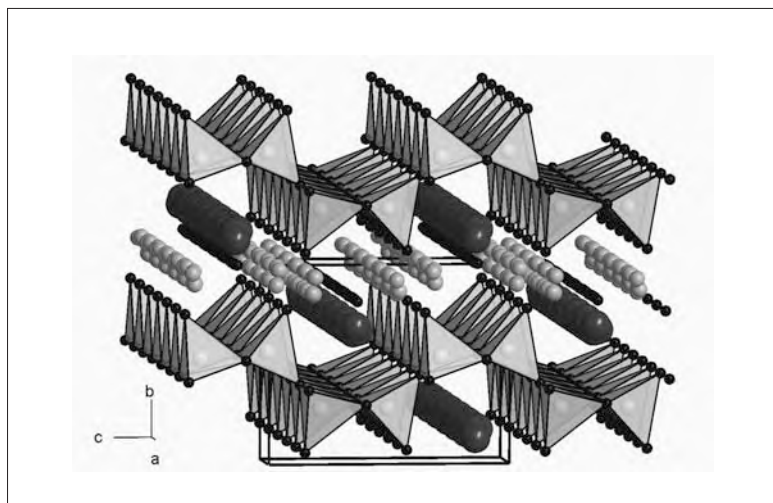
Abb. 4. Die Kristallstruktur des grün leuchtenden Sialons \text{Sr}_5\text{Al}_{5+x}\text{Si}_{21-x}\text{N}_{35-x}\text{O}_{2+x}:\text{Eu}^{2+} ( x \approx 0 ). 12)
