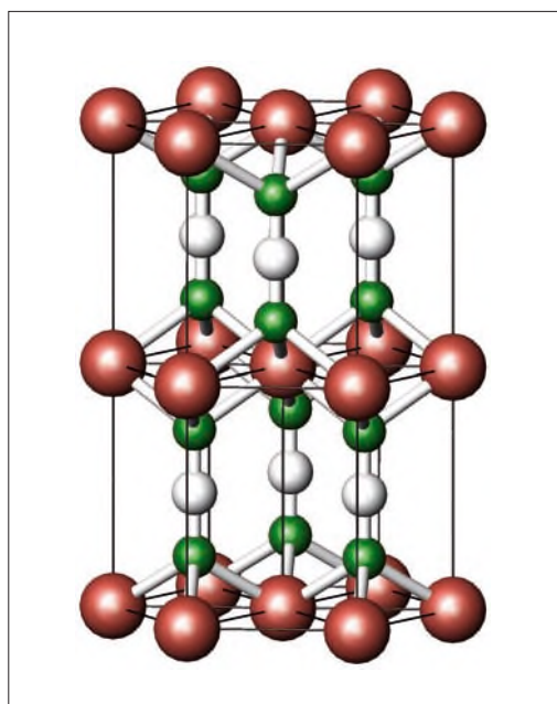
Abb. 5. Kristallstruktur von Fe(NCN). 14)
