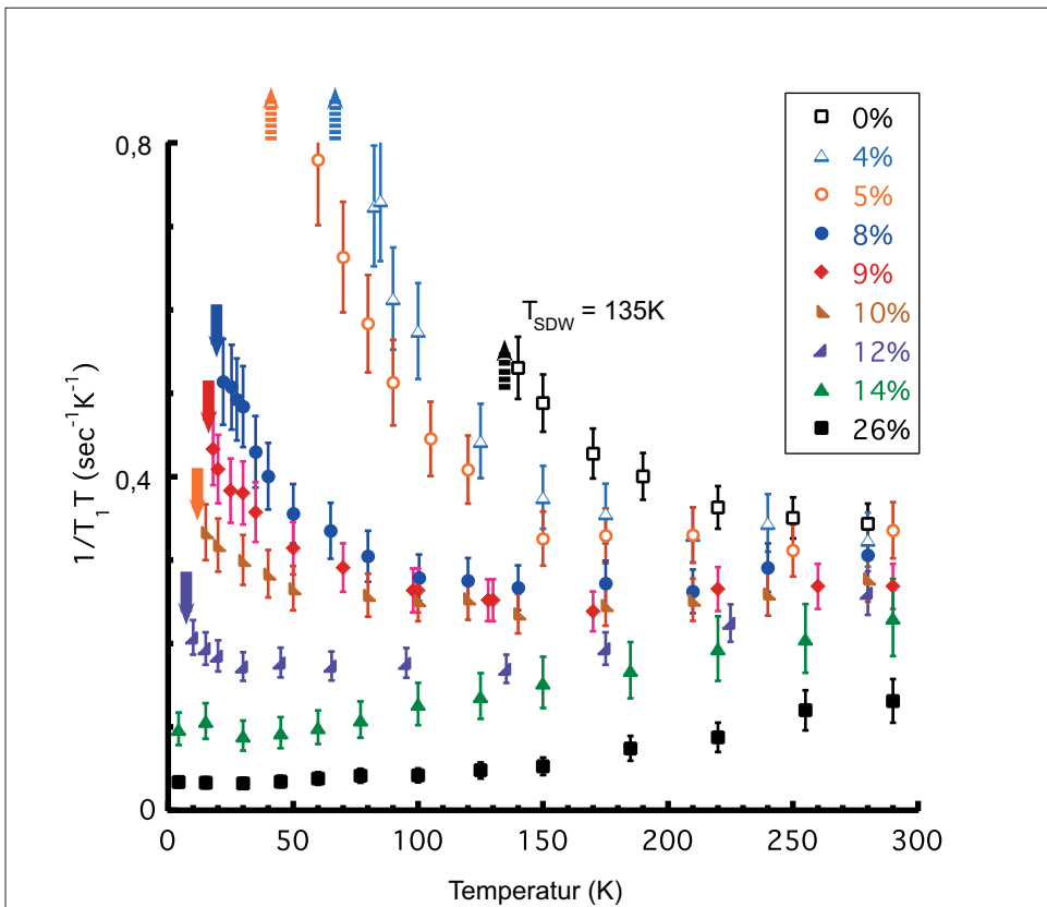
Abb. 3. Spinfluktuationen in Eisenpnictidsupraleitern, bestimmt aus der Spin-Gitter-Relaxationsrate von ^{75}\text{As} -NMR-Resonanzen; 10) mit zunehmender Dotierung beobachtet man, wie zunächst Spinfluktuationen durch Ausbilden der Spindichtewelle stärker werden, bei höherer Dotierung und niedriger Temperatur kollabiert die Spindichtewelle, und damit nimmt auch das Produkt aus Relaxationsrate und inverser Temperatur ab.
