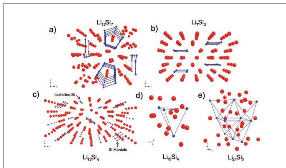
Abb. 14. Die Strukturen der verschiedenen Li-Si-Legierungen, die während des Einbaus von Li in Si auftreten. 33)
