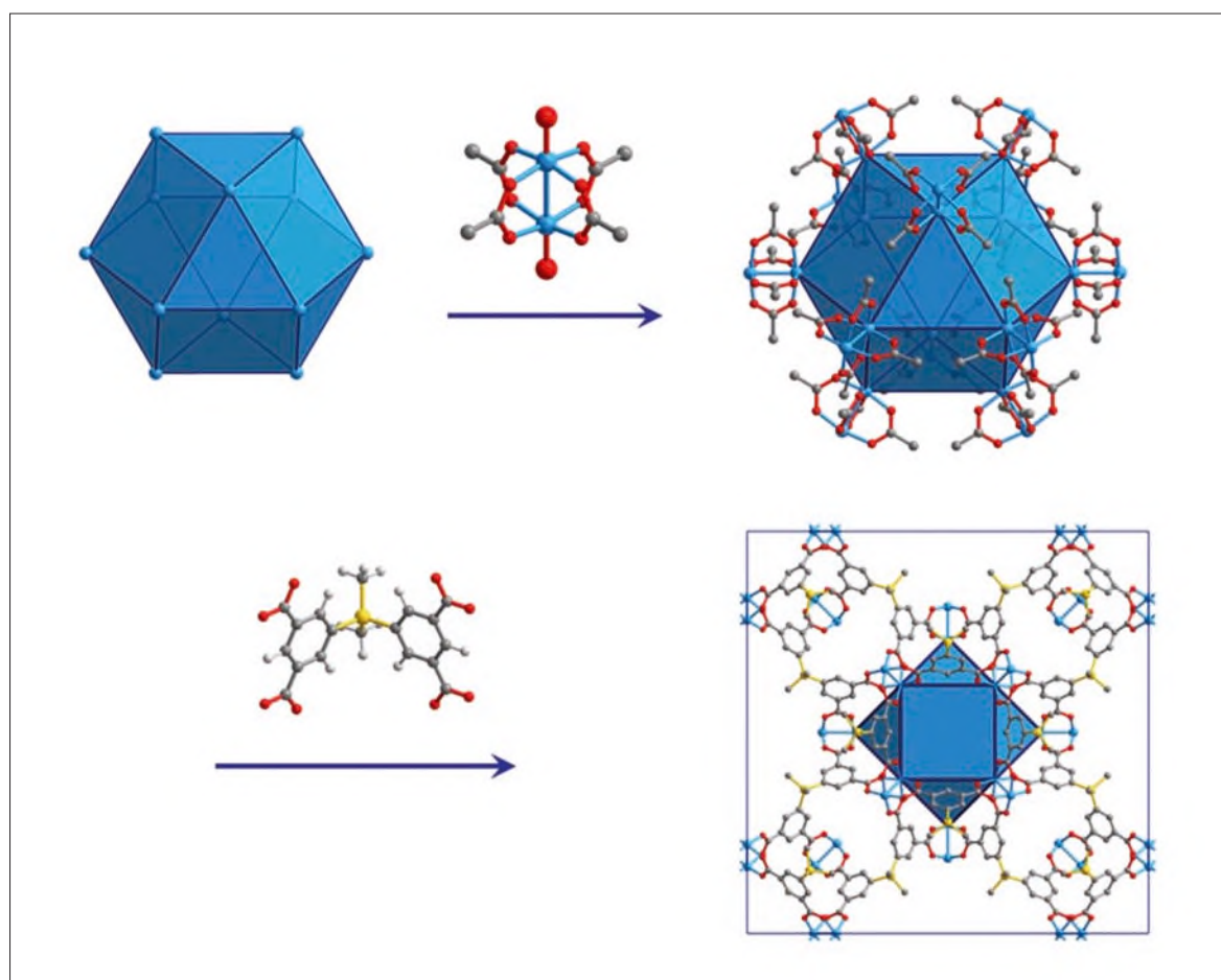
Abb. 11. Der Aufbau von PCN-12-Si: Di-Kupfer-Schaukelrad-Einheiten als sekundäre Baugruppen besetzen die Ecken eines Kuboktaeders, während 24 Isophtalatgruppen die Kanten bilden. 26) Unten rechts ist die gesamte Einheitszelle entlang der c -Achse abgebildet.
