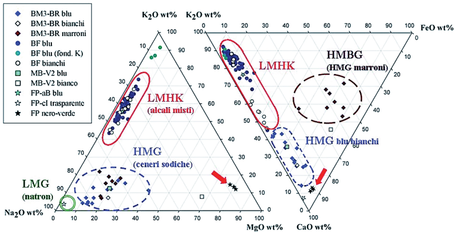
Fig. 3 – Diagrammi ternari Na 2 O-MgO-K 2 O e FeO-K 2 O-CaO. Si evidenziano le diverse aree composizionali. Sono diagrammati per confronto anche dati di letteratura relativi a vetri dell'Italia Settentrionale del BM3 – BF (da Angelini 2009; Angelini et al. 2002, 2004, 2005 e 2009; e letteratura citata).
