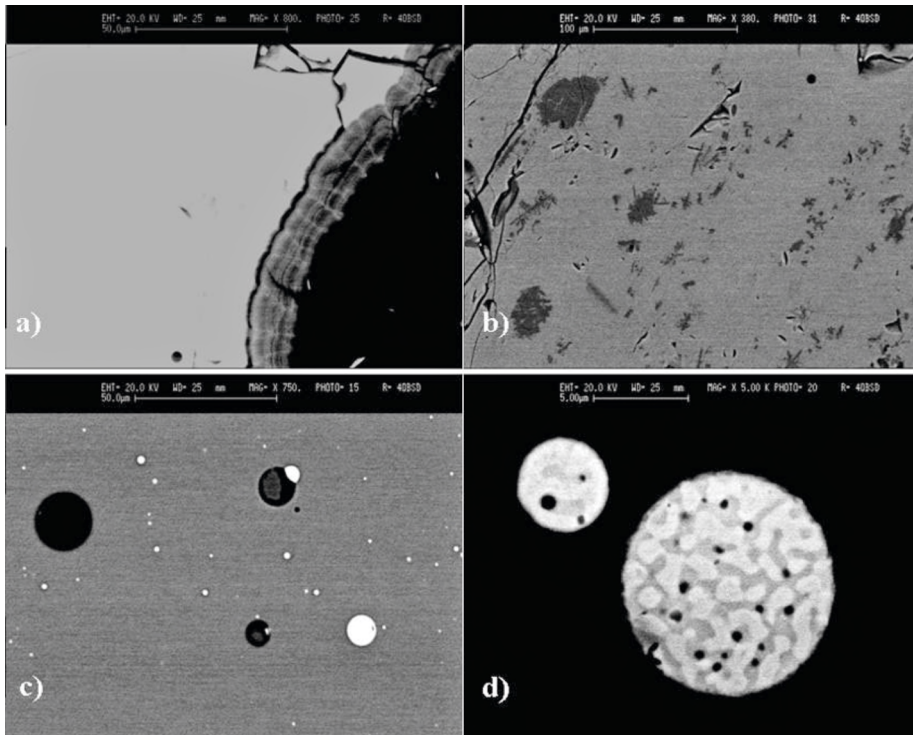
Fig. 2 – Immagini SEM-BSE dei campioni: a) Vetro blu omogeneo di MB-V2, con strato di alterazione (grigio scuro); b) fase vetrosa di FP-aB in cui si vedono inclusioni di \text{SiO}_2 (grigio scuro); c) campione FP-bV, visibili bolle di diverse dimensioni (nere) e segregazioni di Fe-P-S (bianche); d) campione FP-bN, particolare di una segregazione zonata di Fe-P-S: aree grigie alto P, aree nere alto S.
