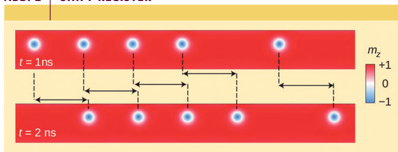
ABB. 2 | SHIFT-REGISTER
